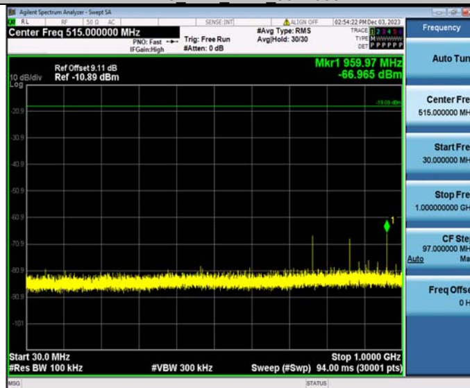
DH5 Ant1 2441 30~1000
