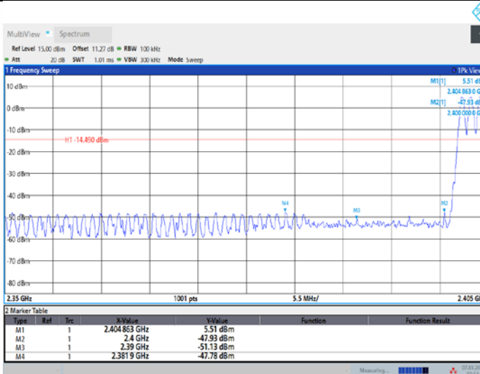
DH5_Ant1_Low_Hop_2402
