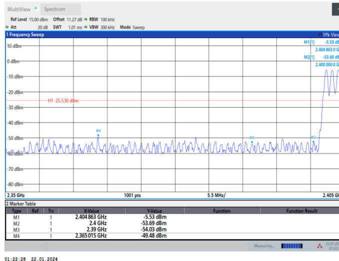
DH5_Ant1_Low_Hop_2402
