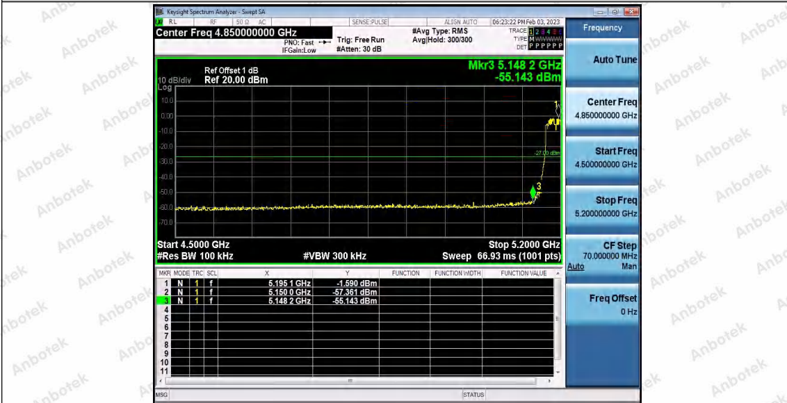
11AX40SISO_Ant2_Low_5190
