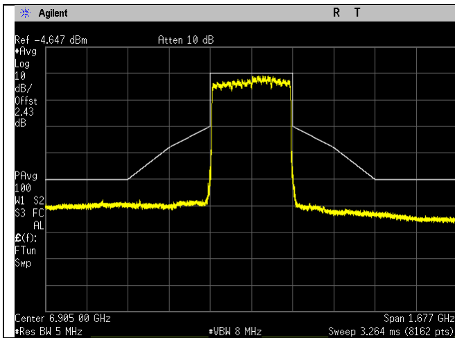
6905MHz_191_320MHz BW_be-mode_Chain 0
