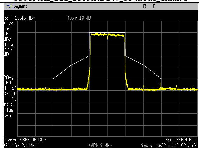
6665MHz_143_160MHz BW_be-mode_Chain 1
