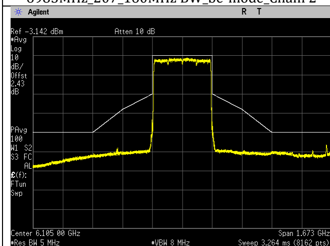
6105MHz_31_320MHz BW_be-mode_Chain 0
