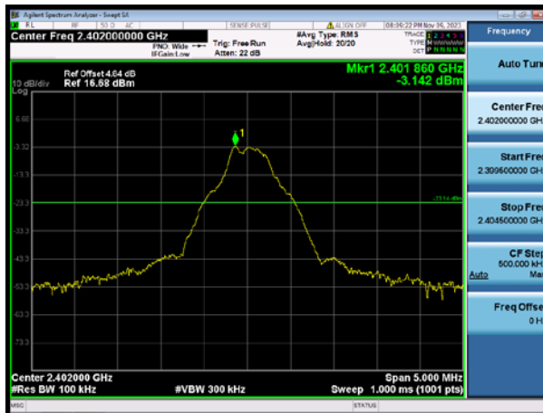
GFSK 2402MHz
