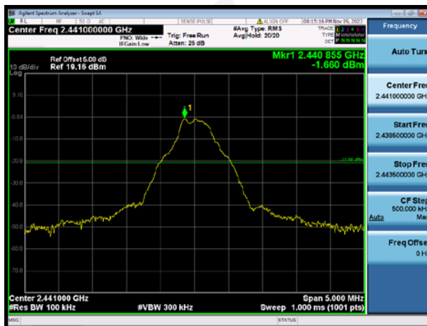
GFSK 2441MHz
