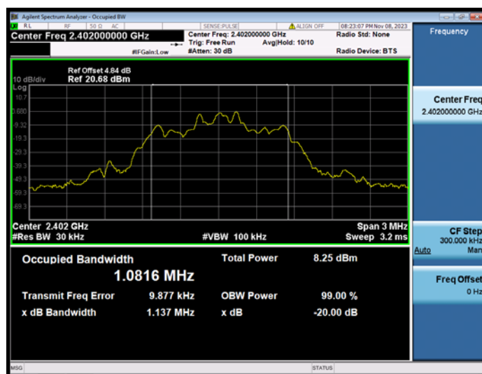
\pi/4 -DQPSK (2-DH1) 2402MHz
