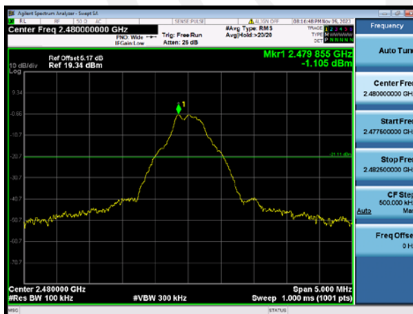
GFSK 2480MHz
