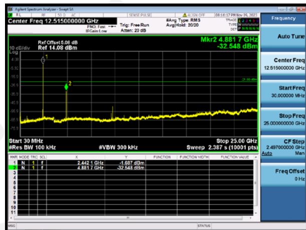
GFSK 2441MHz
