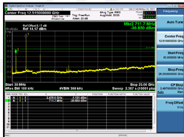
GFSK 2480MHz
