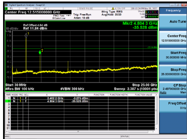
GFSK 2402MHz
