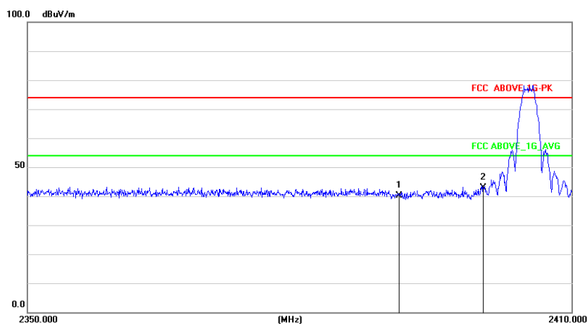
2405MHz Vertical
