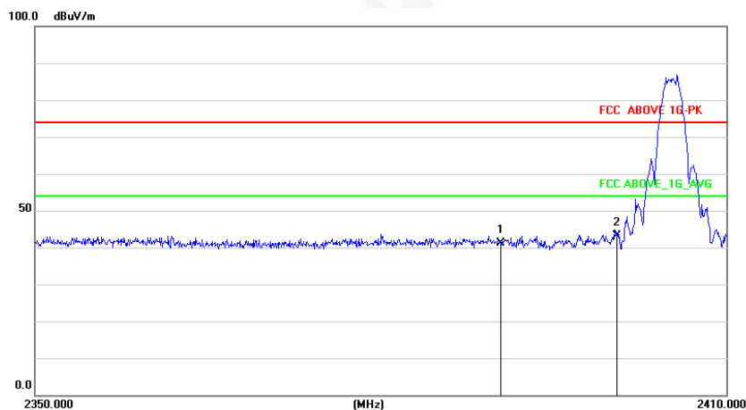
2405MHz Horizontal
