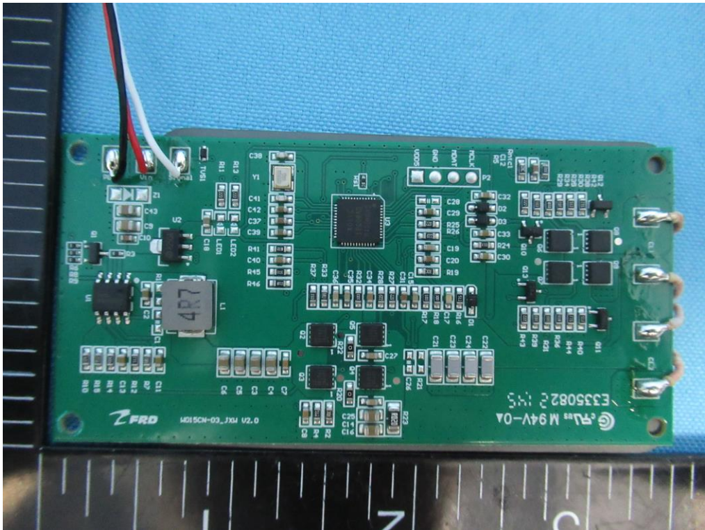
(3) EUT Photo
