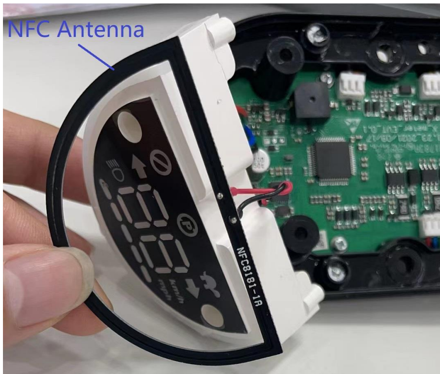
(6) EUT Photo
