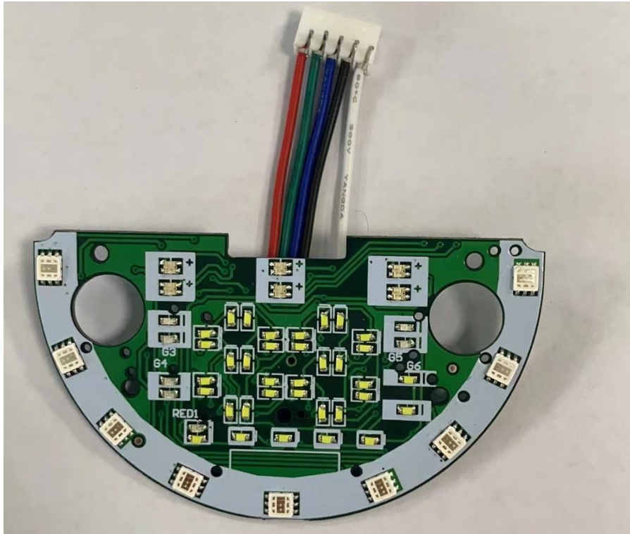
(9) EUT Photo
