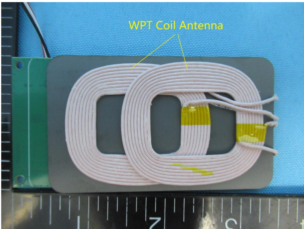
(4) EUT Photo
