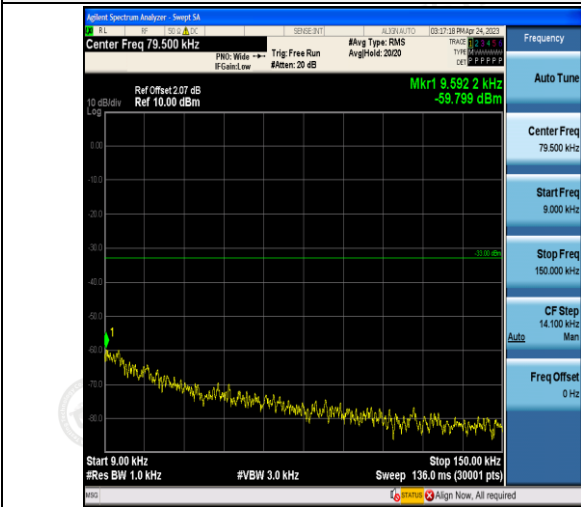
0.009~0.15MHz
