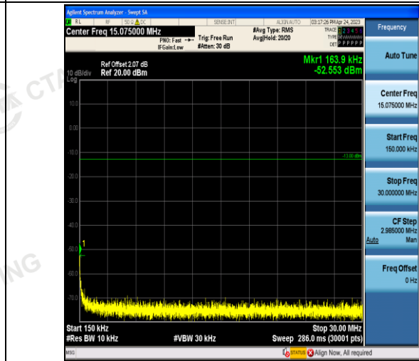
0.15~30MHz
