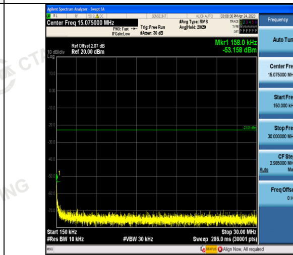
0.15~30MHz
