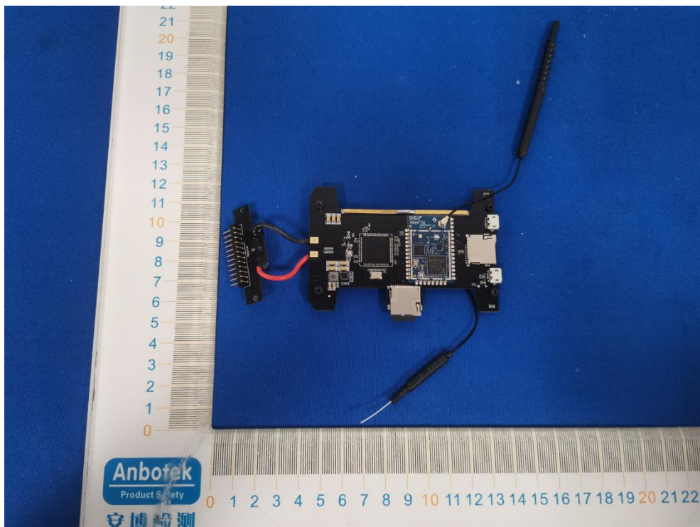
915MHz ANT
