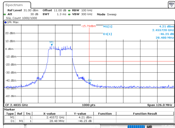
n20_2462MHz_Chain 0
