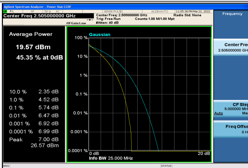
Band7-10MHz-QPSK-20800-50RB#0
