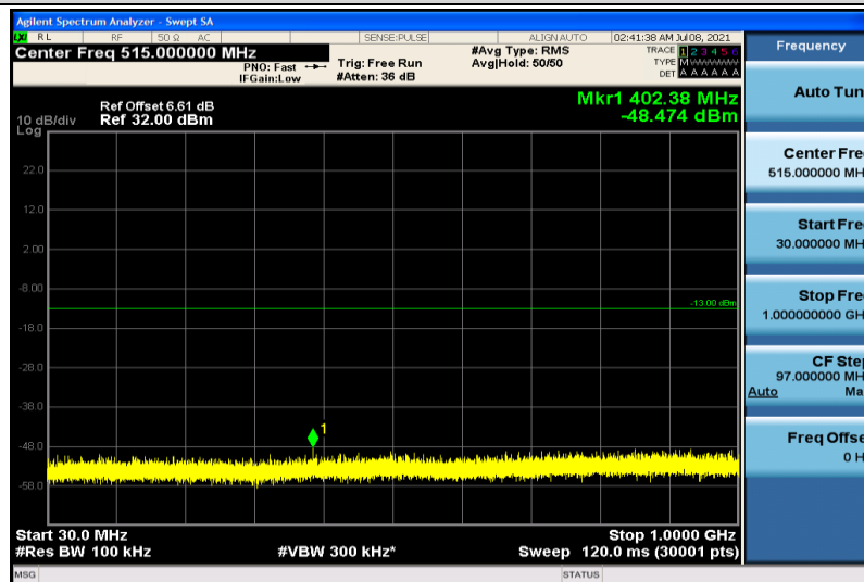
Band4-3MHz-QPSK-20385-1RB#0-30~1000MHz
