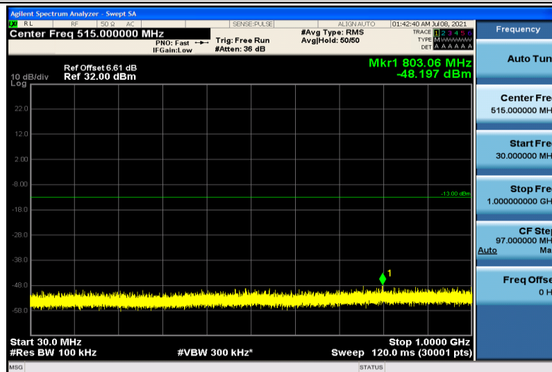
Band2-20MHz-16QAM-19100-1RB#0-30~1000MHz
