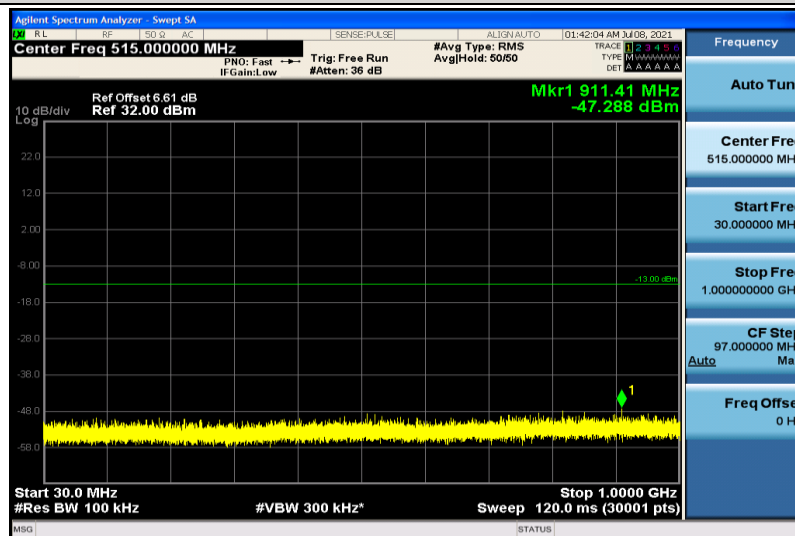
Band2-20MHz-QPSK-19100-1RB#0-30~1000MHz
