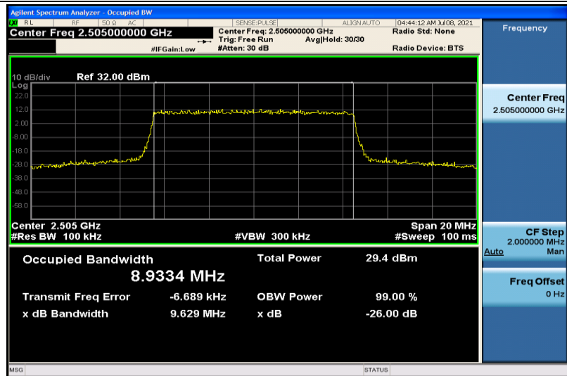
Band7-10MHz-QPSK-20800-50RB#0-8.9334
