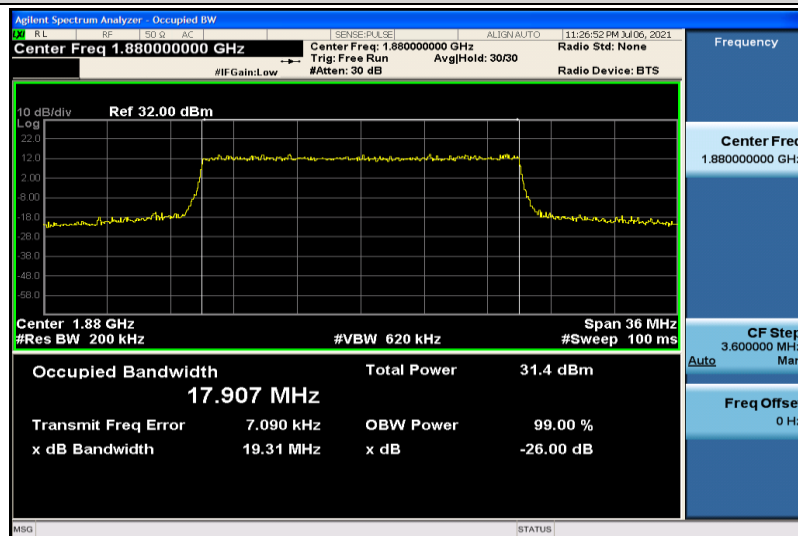
Band2-20MHz-QPSK-18900-100RB#0-17.907
