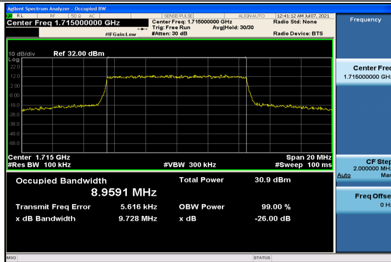
Band4-10MHz-QPSK-20000-50RB#0-8.9591
