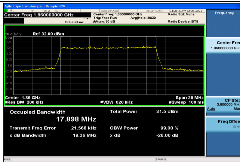
Band2-20MHz-QPSK-18700-100RB#0-17.898
