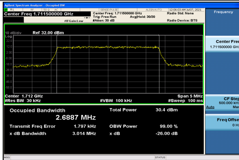
Band4-3MHz-QPSK-19965-15RB#0-2.6887
