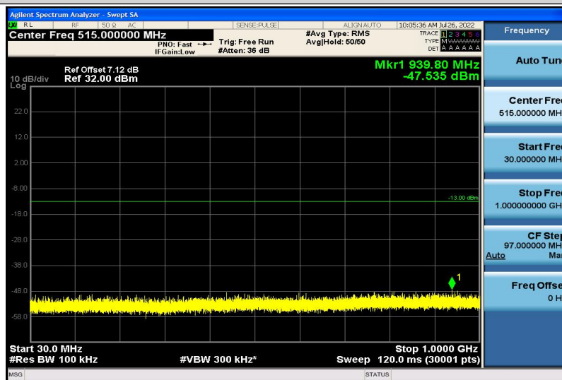
Band2-3MHz-QPSK-18900-1RB#0-30~1000MHz
