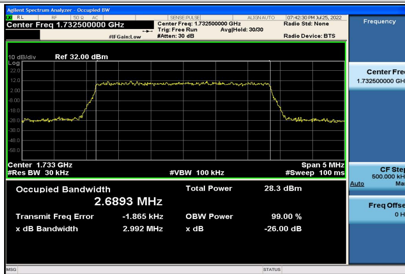
Band4-3MHz-QPSK-20175-15RB#0-2.6893
