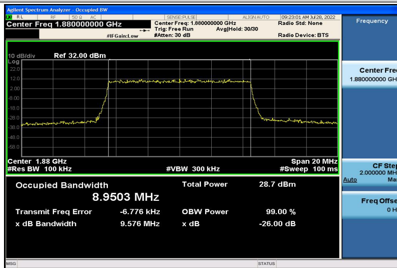
Band2-10MHz-QPSK-18900-50RB#0-8.9503
