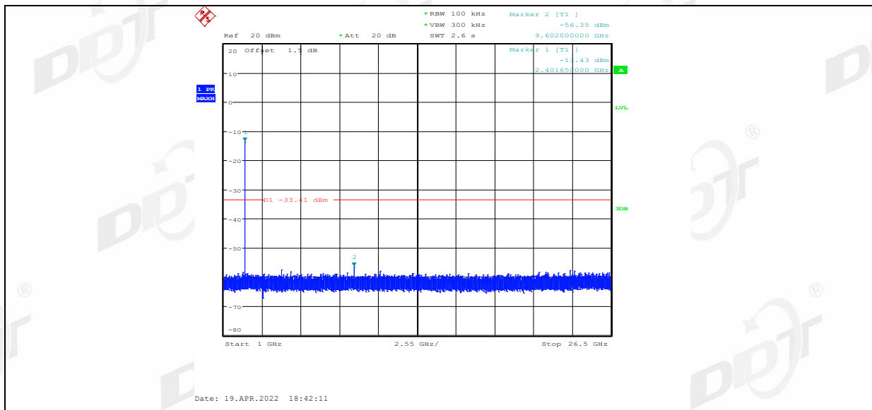
BLE 1M_Ant1_2440_0~Reference
