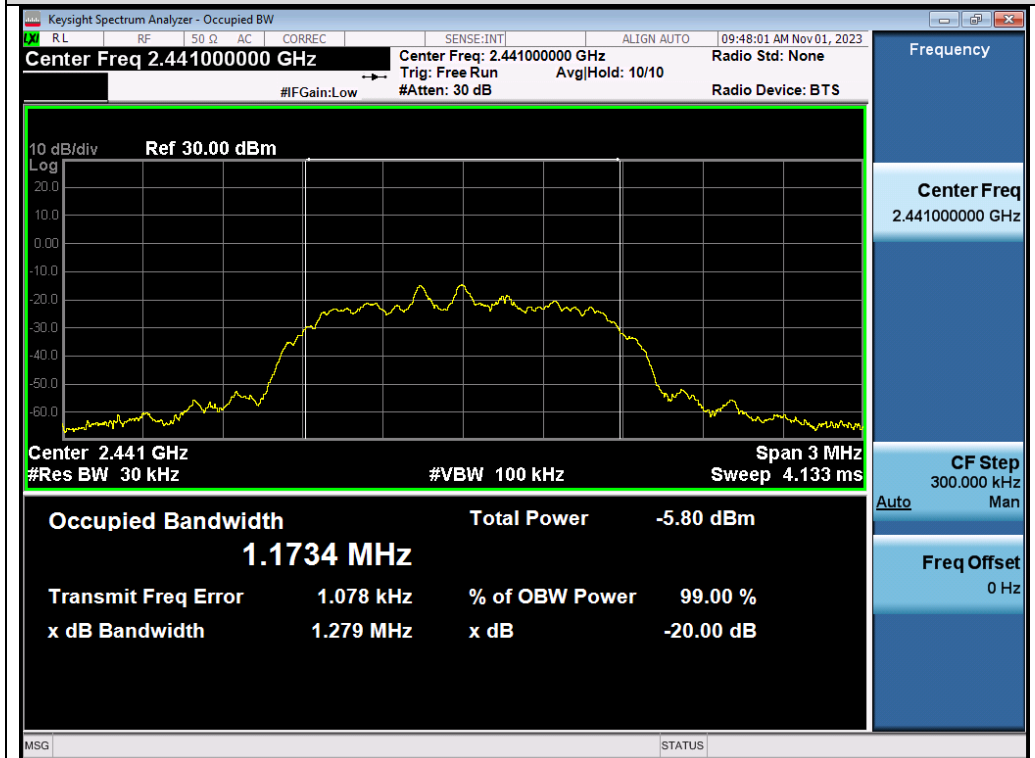
Test_Graph_π /4-DQPSK_ANT1_2441_OBW
