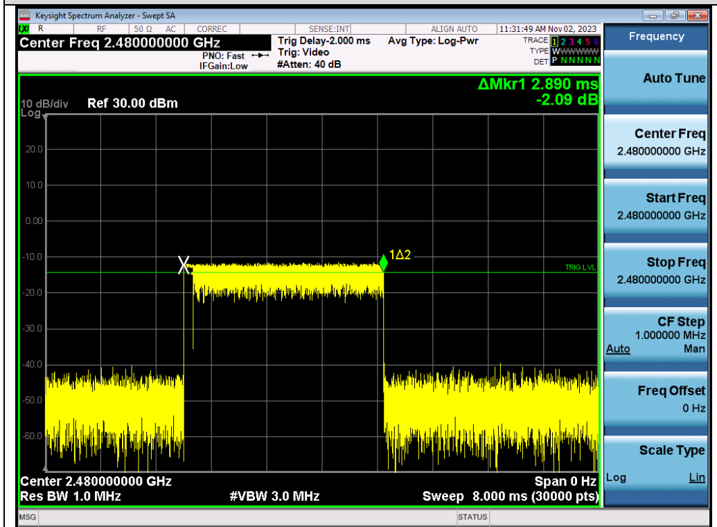
Test_Graph_π /4-DQPSK_HOP_ANT1_NA_1Mbps_2480_Time per Burst
