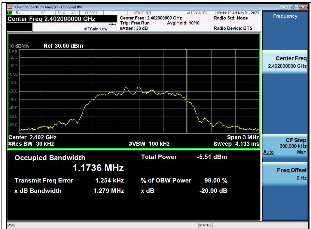
Test_Graph_π /4-DQPSK_ANT1_2402_OBW
