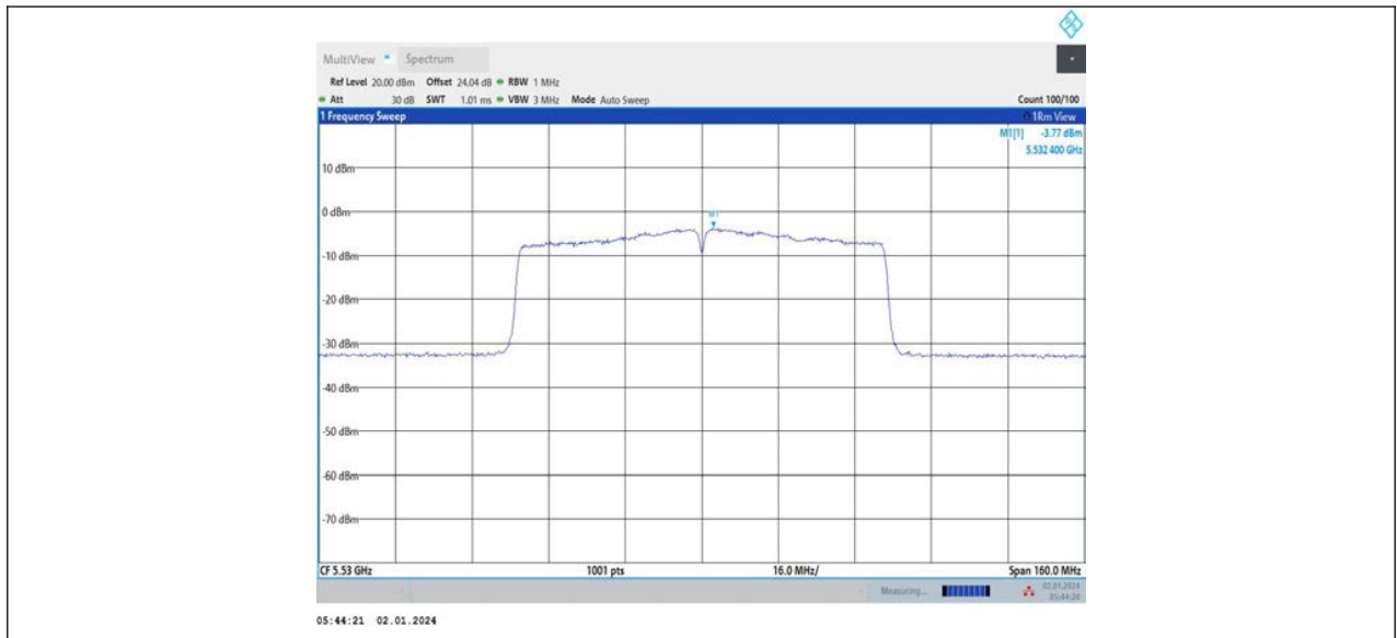
11AC80MIMO_Ant2_5530
