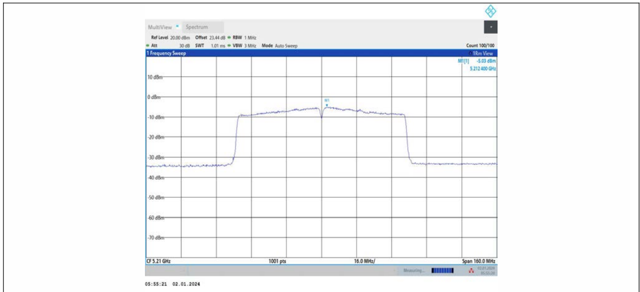
11AC80MIMO_Ant2_5210
