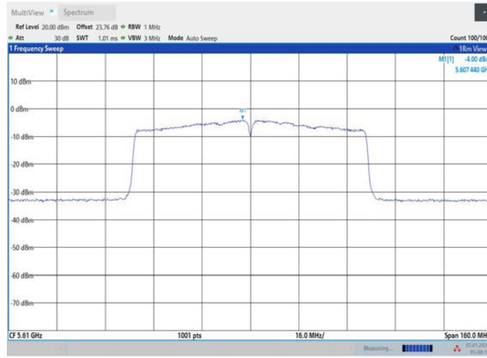
11AC80MIMO_Ant2_5610
