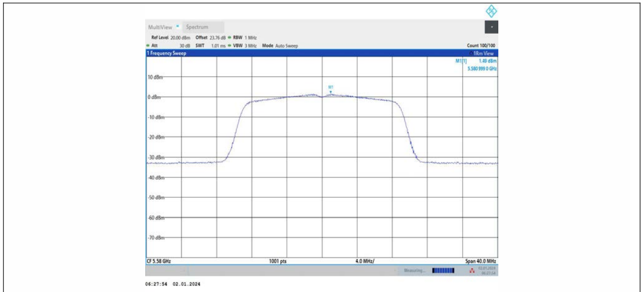
11AC20MIMO_Ant2_5580
