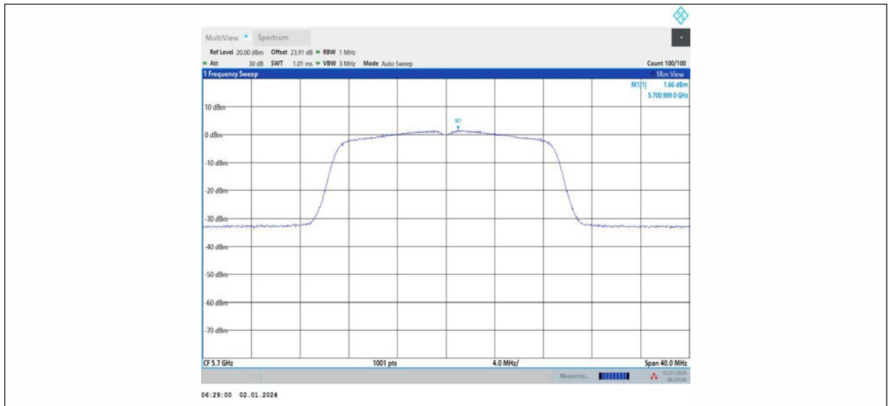
11AC20MIMO_Ant2_5700
