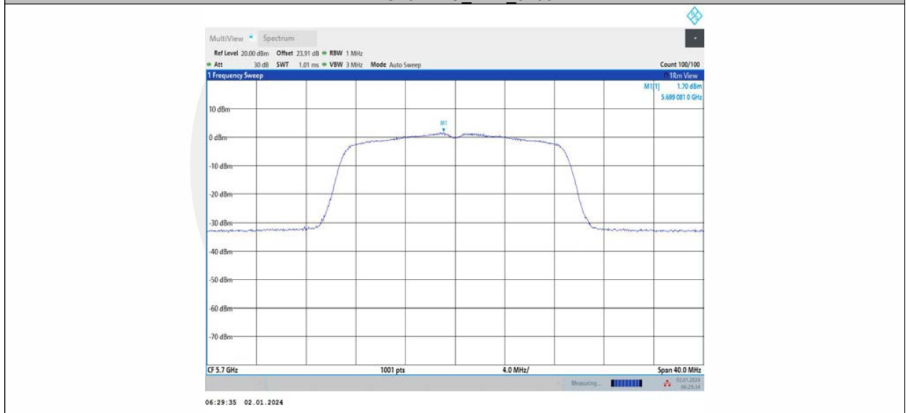
11AC20MIMO_Ant1_5745
