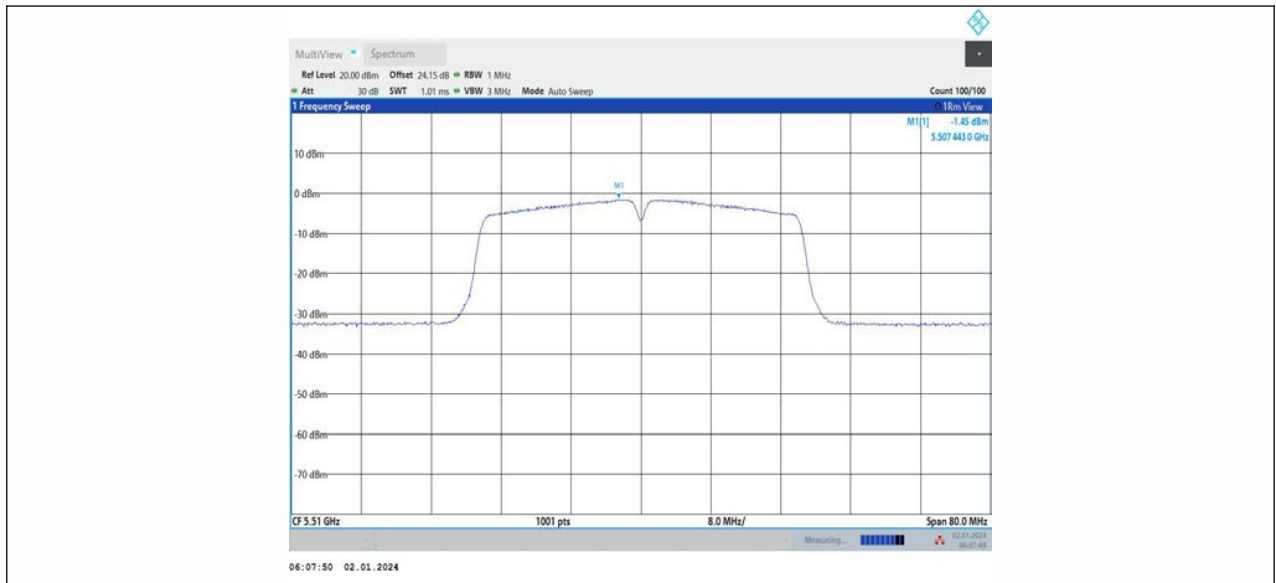
11AC40MIMO_Ant2_5510
