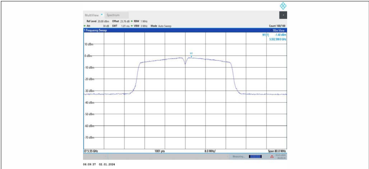
11AC40MIMO_Ant2_5550
