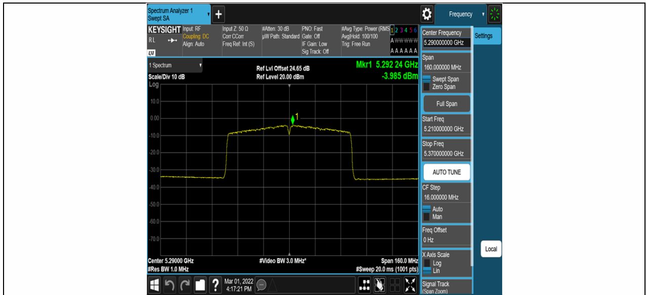
11AC80SISO_Ant2_5290
