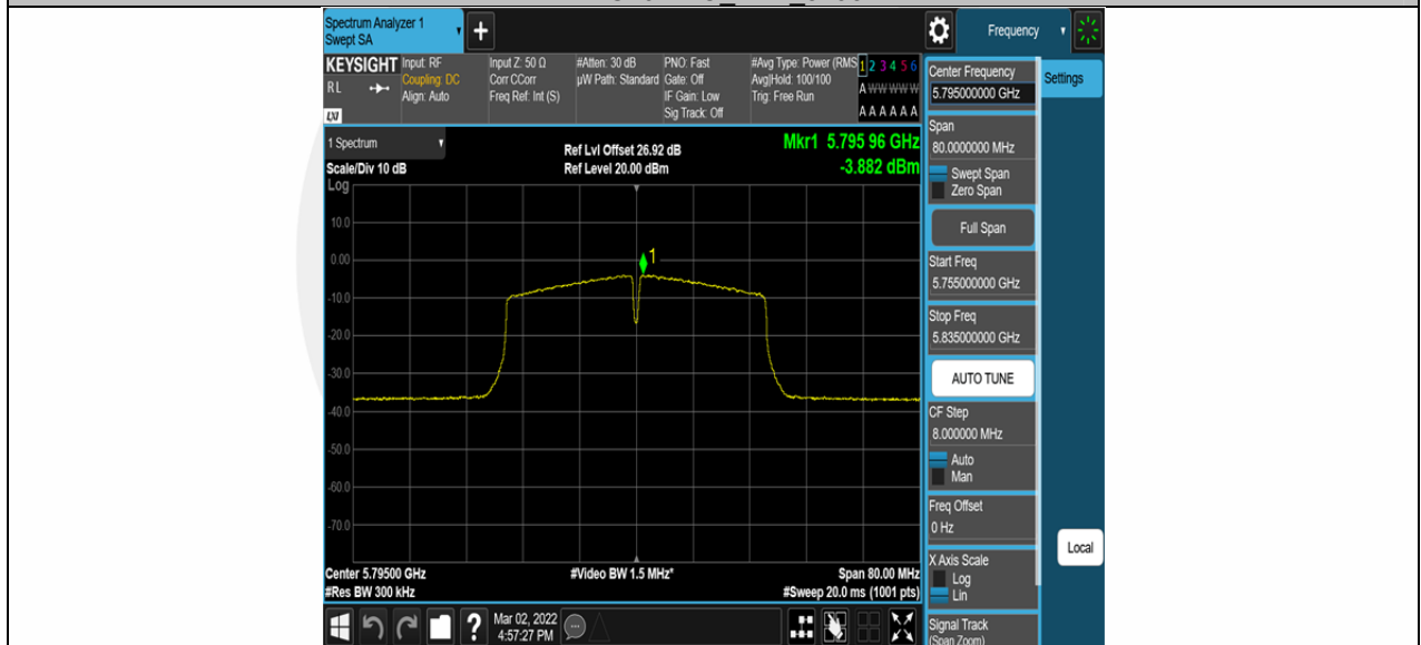
11AC80SISO_Ant1_5210
