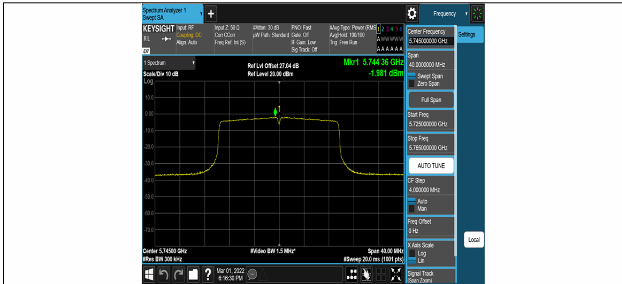
11AX20SISO_Ant2_5745
