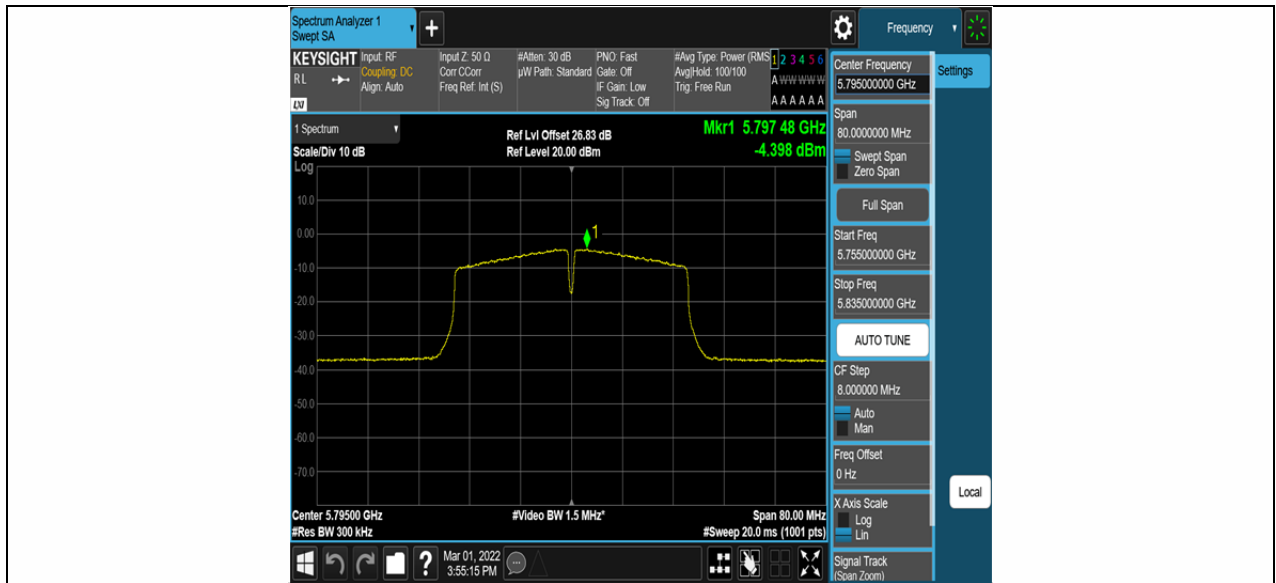
11AC40SISO_Ant2_5795
