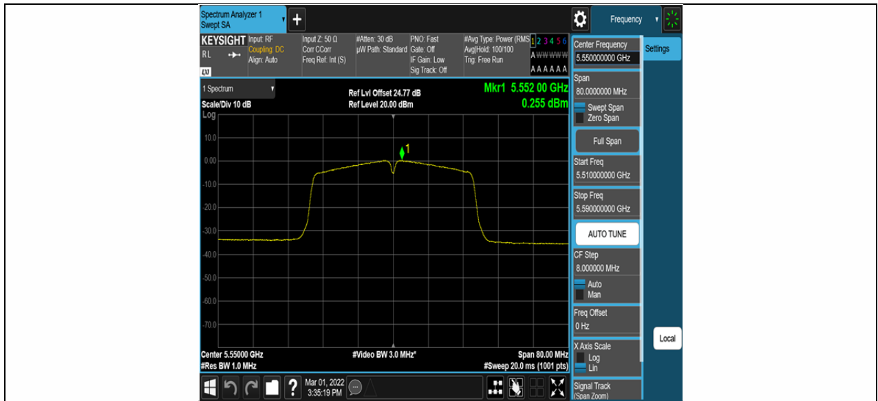
11AC40SISO_Ant2_5550
