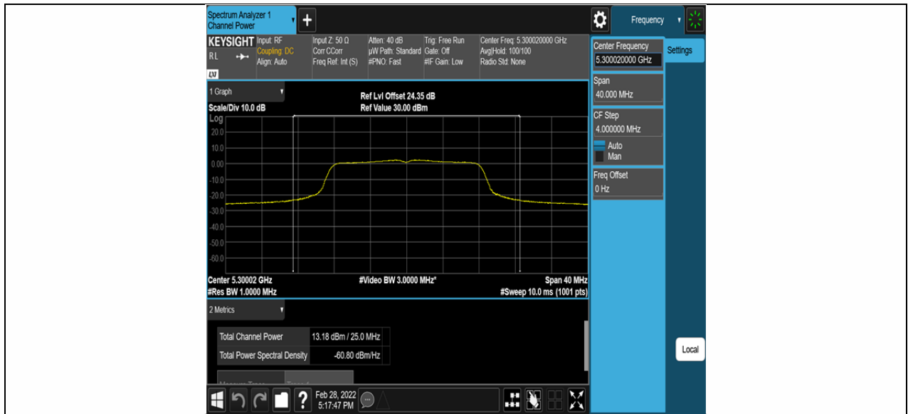
11A_Ant2_5300
