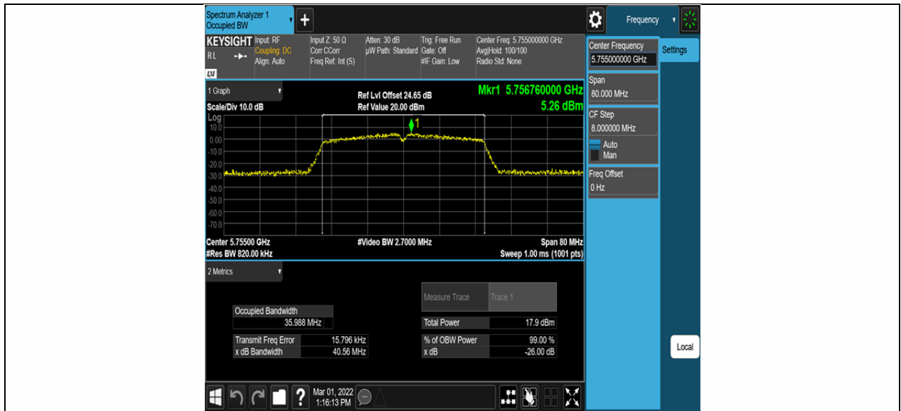
11N40SISO_Ant2_5755
