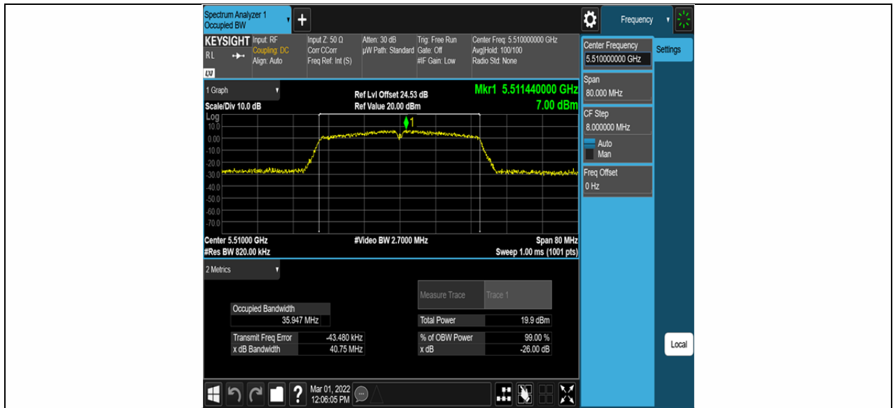
11N40SISO_Ant2_5510
