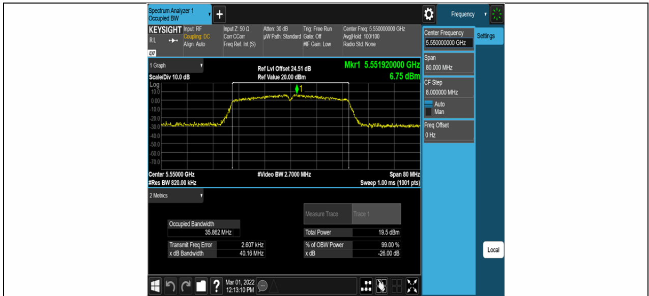
11N40SISO_Ant2_5550
