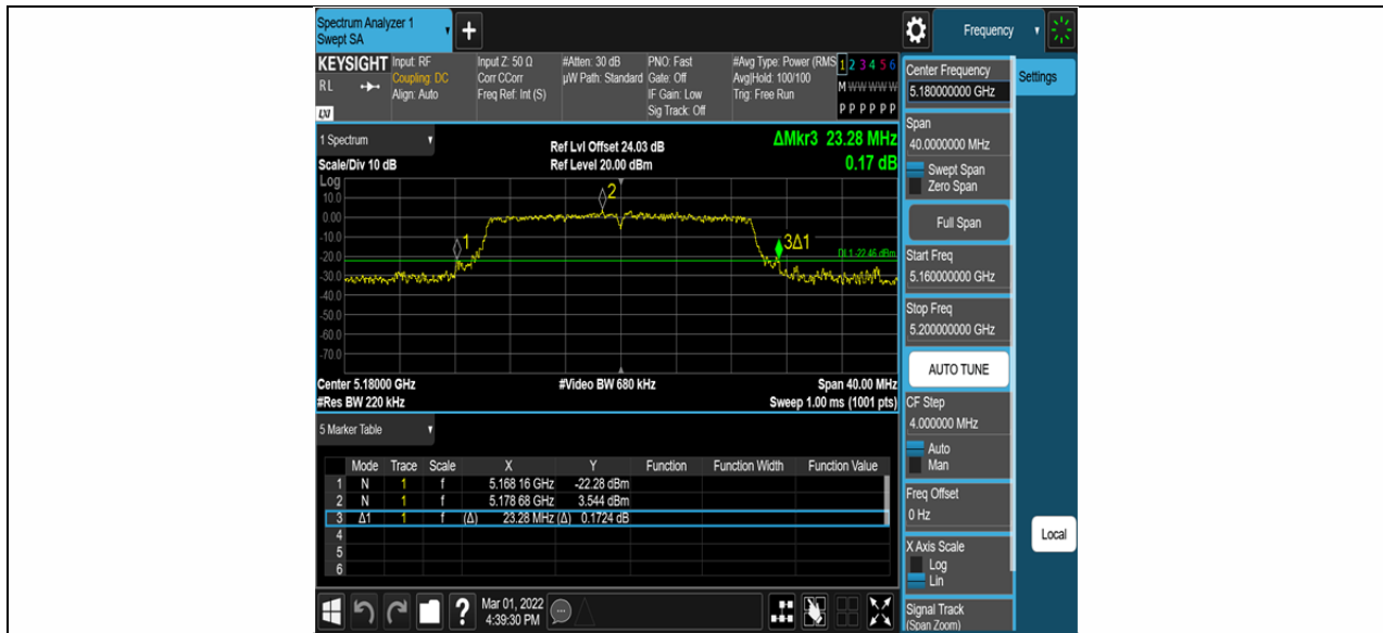
11AX20SISO_Ant2_5180
