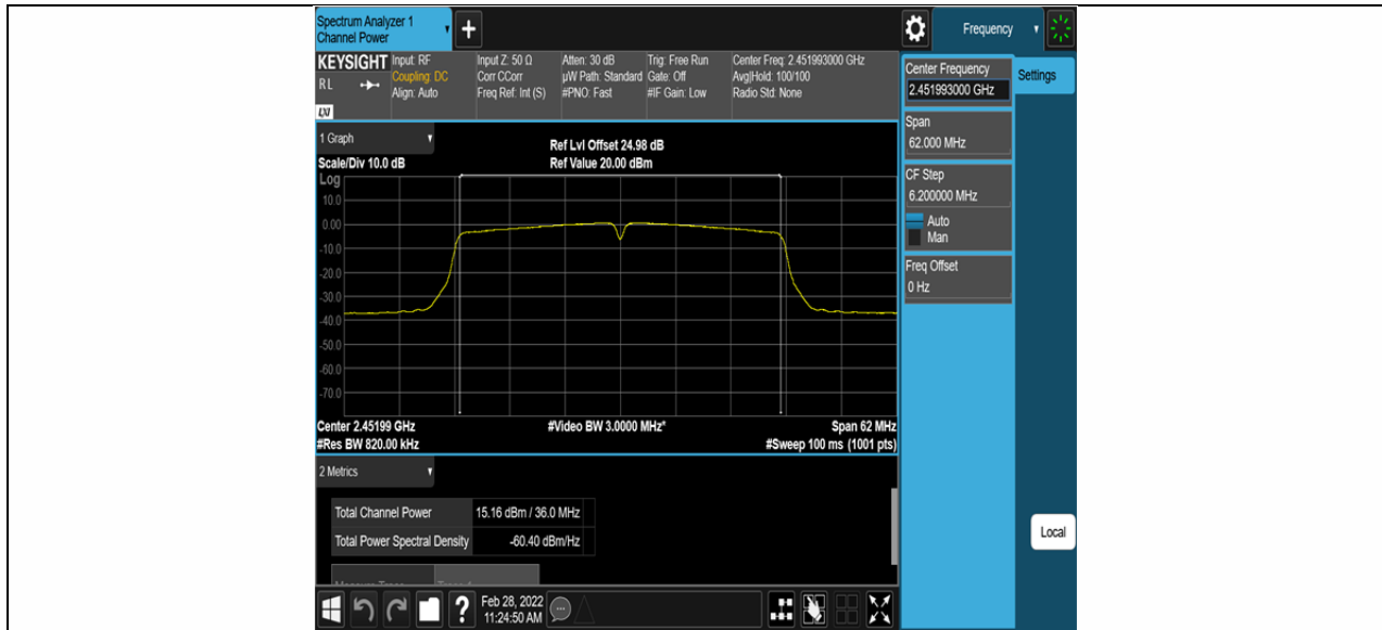
11N40SISO_Ant2_2452
