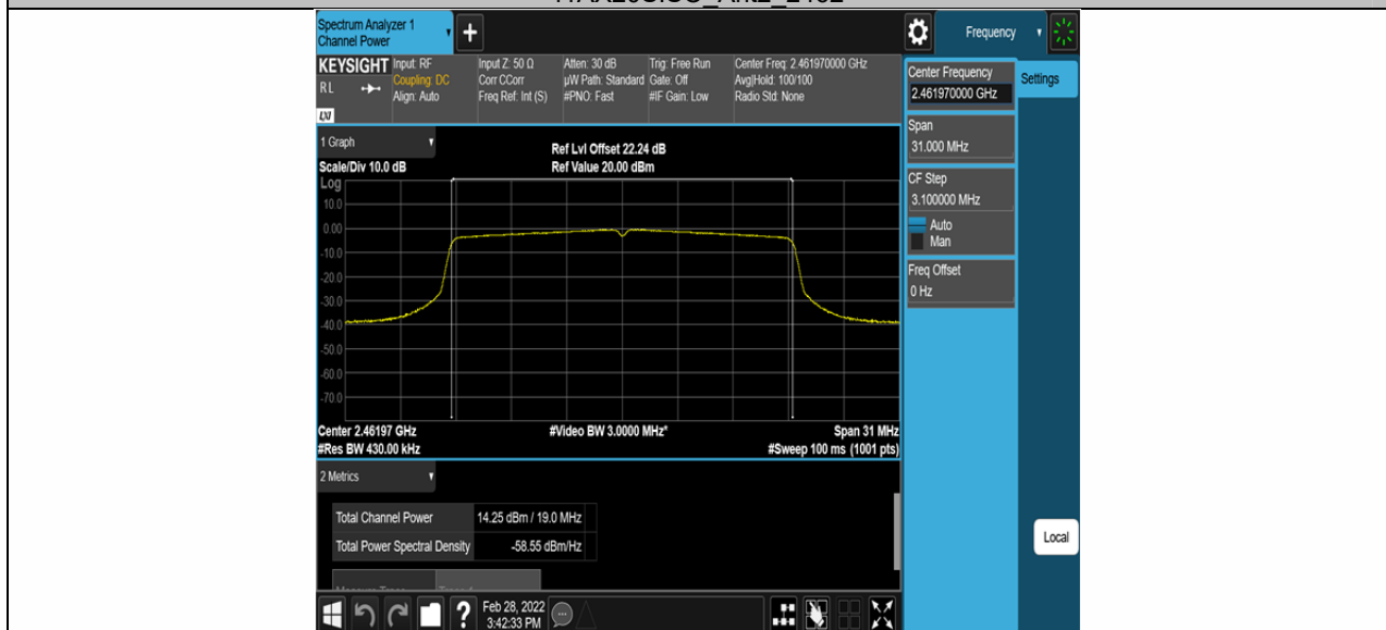
11AX20SISO_Ant2_2462
