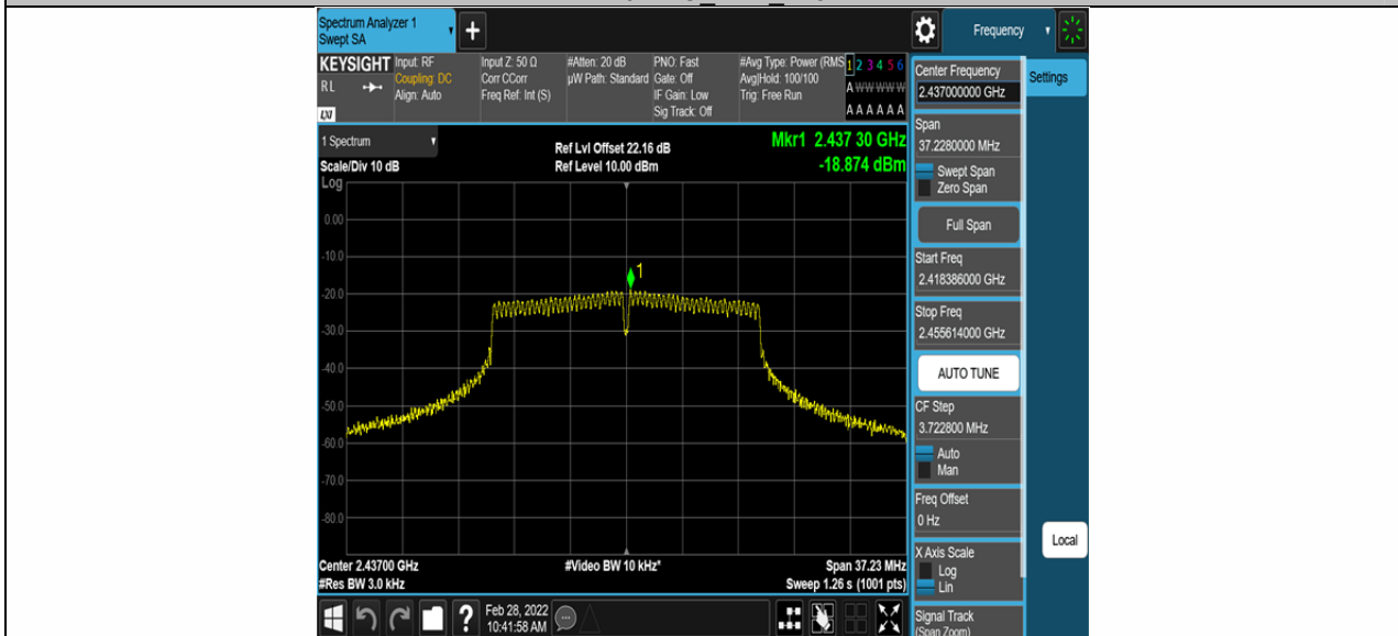
11N20SISO_Ant1_2437
