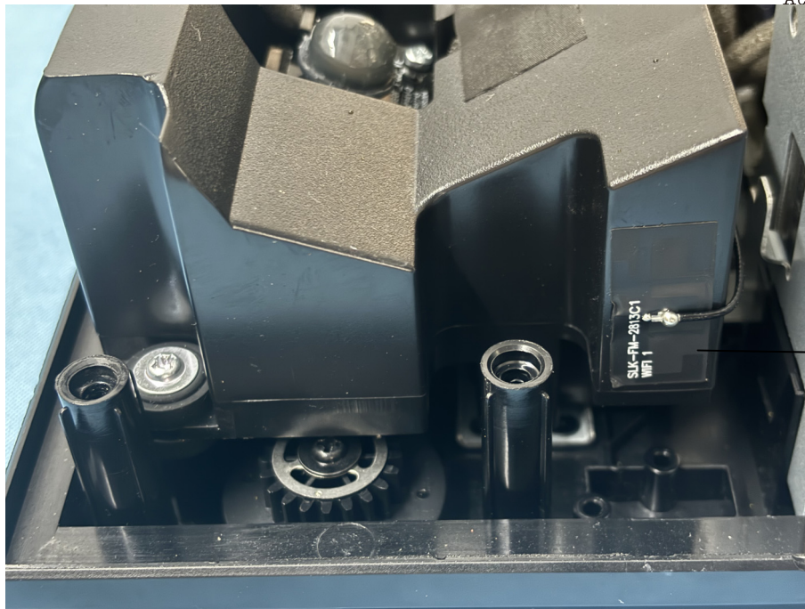
WIFI1 antenna
