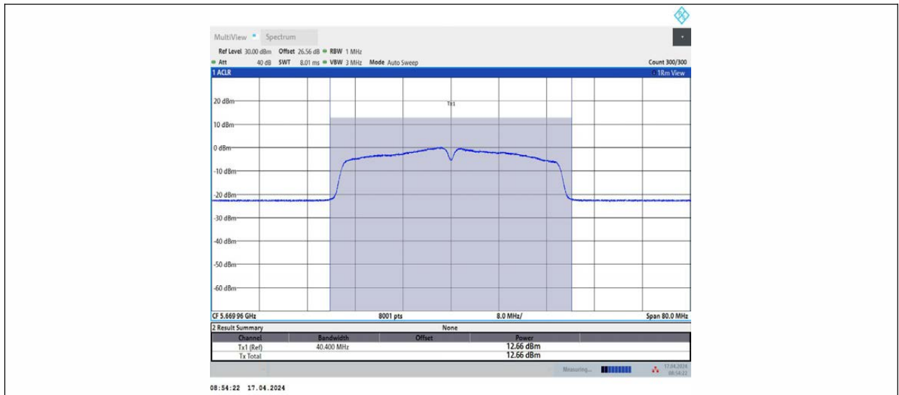
11N40MIMO_Ant2_5670
