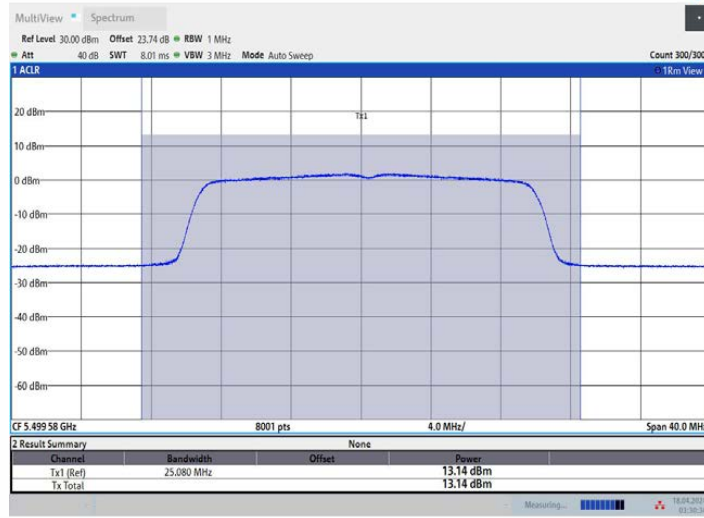
11AX20MIMO_Ant2_5500
