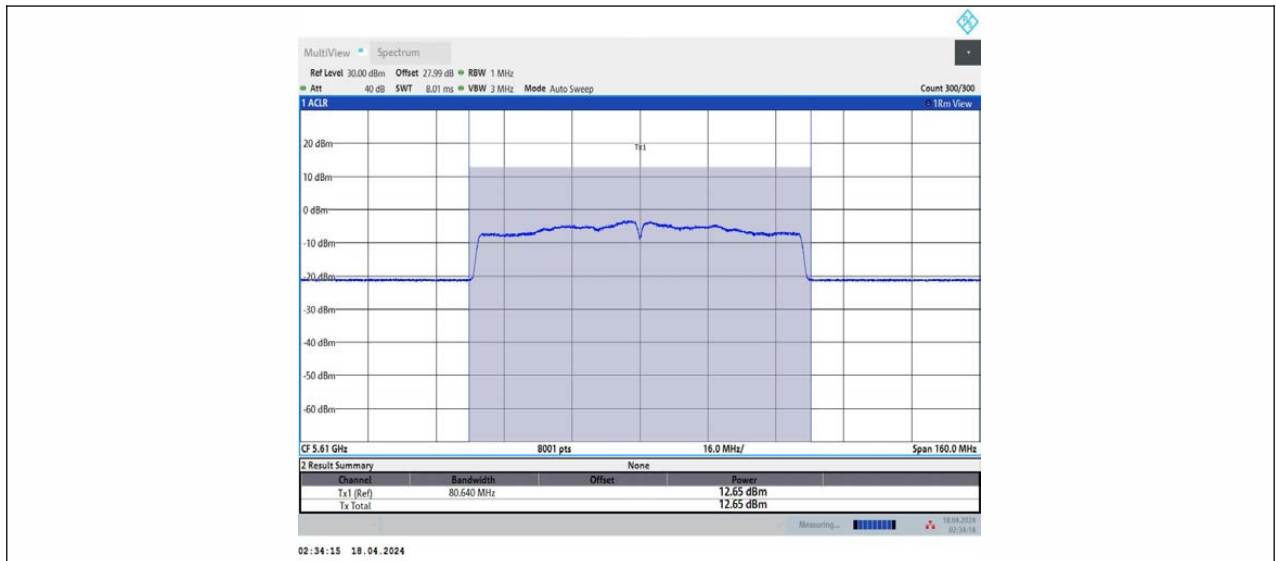
11AC80MIMO_Ant2_5610
