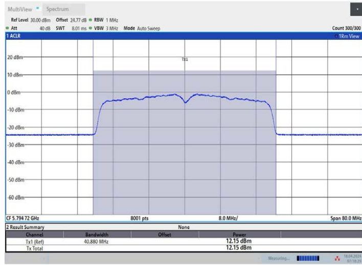
11AX40MIMO_Ant2_5795
