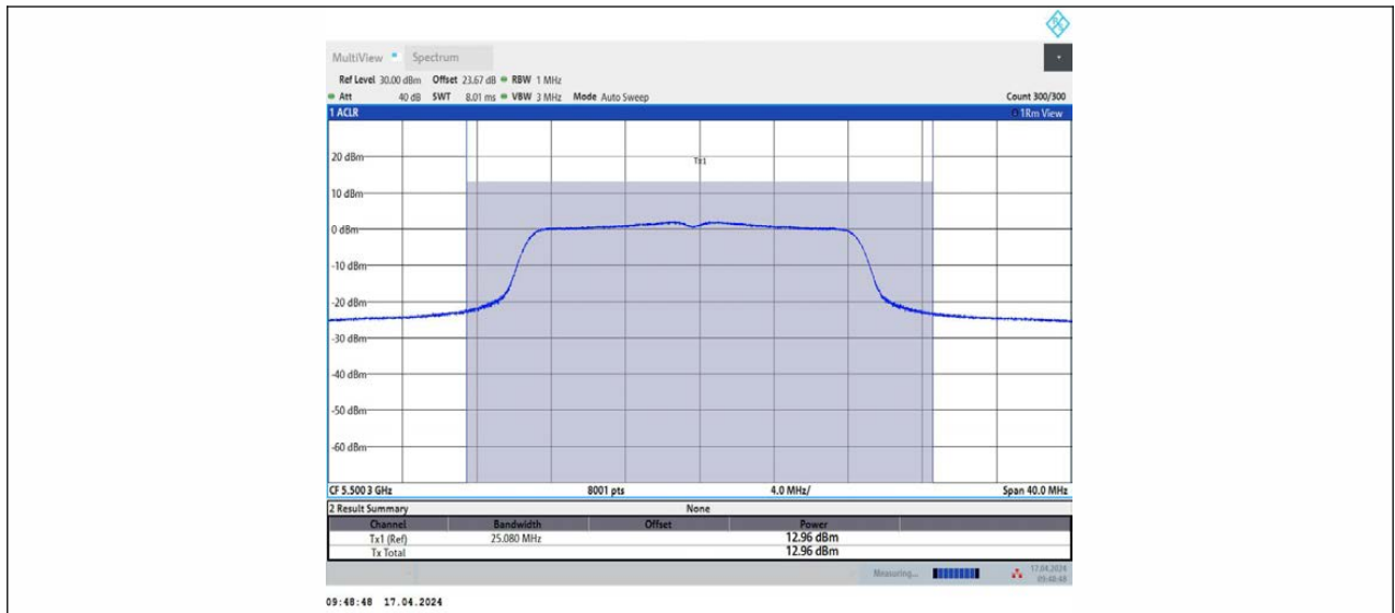
11AC20MIMO_Ant2_5500
