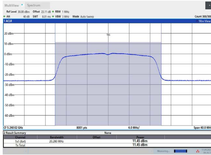
11AC20MIMO_Ant2_5240
