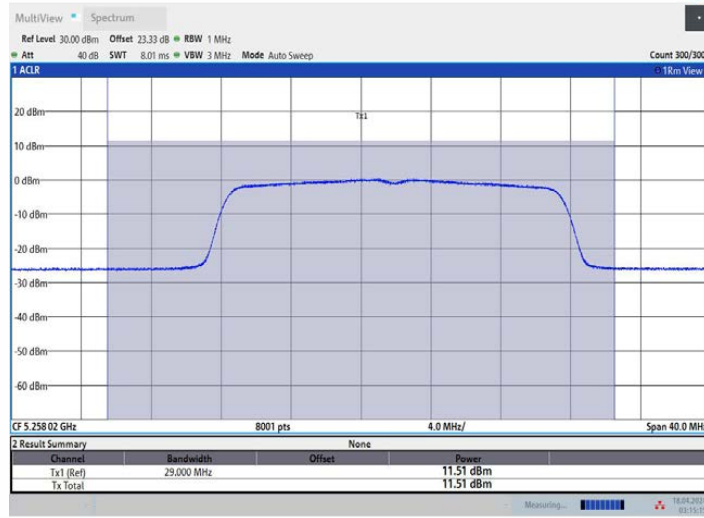
11AX20MIMO_Ant2_5260
