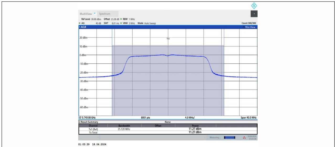
11AC20MIMO_Ant2_5745
