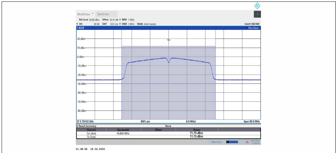
11AC40MIMO_Ant2_5755
