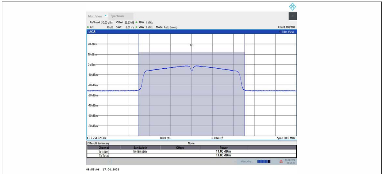
11N40MIMO_Ant2_5755
