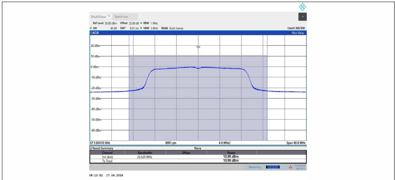
11N20MIMO_Ant2_5825
