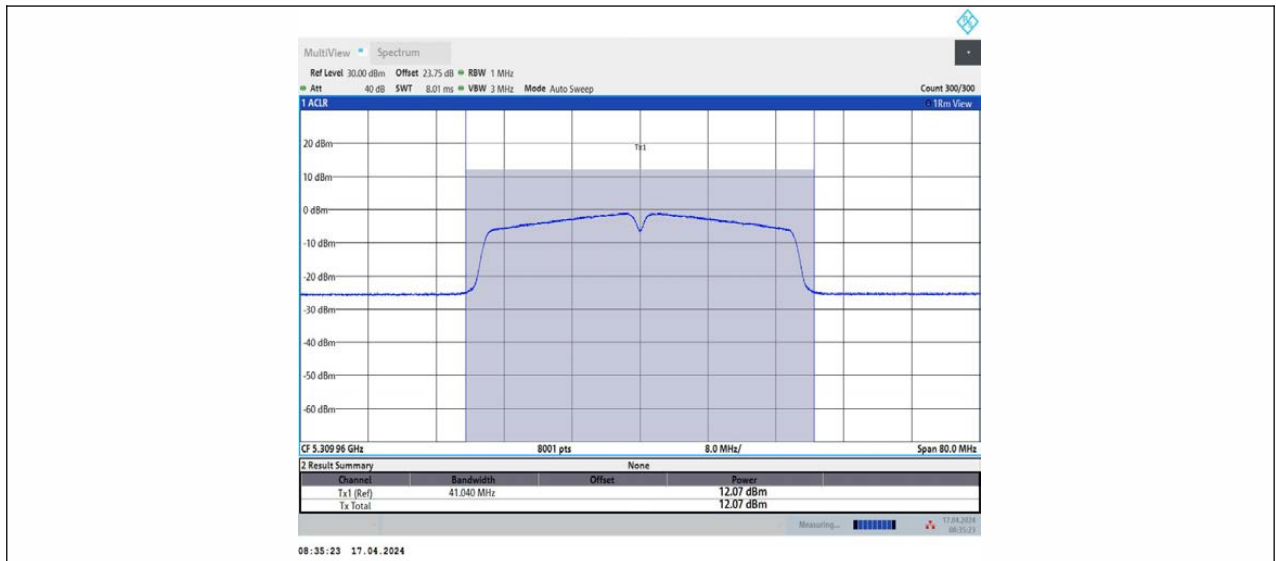
11N40MIMO_Ant2_5310
