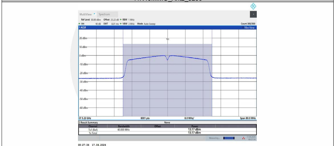
11N40MIMO_Ant1_5270
