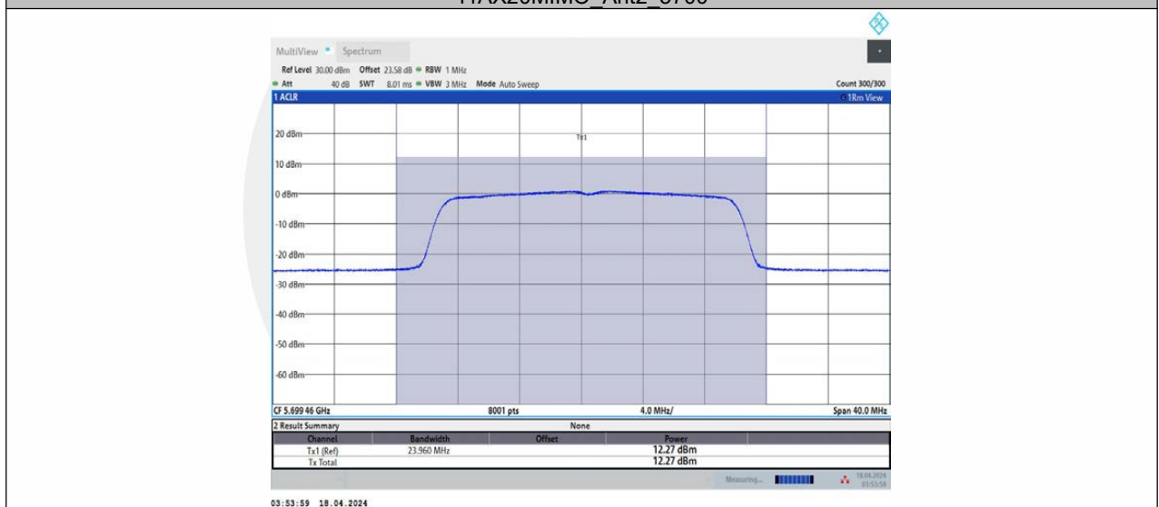
11AX20MIMO_Ant1_5745
