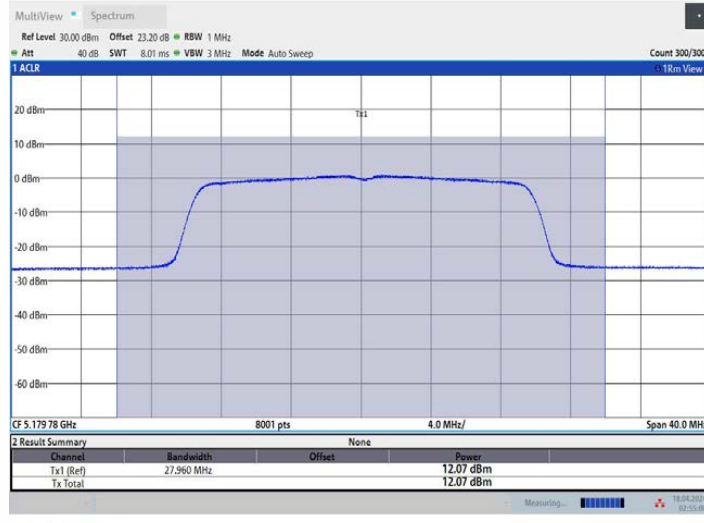
11AX20MIMO_Ant2_5180
