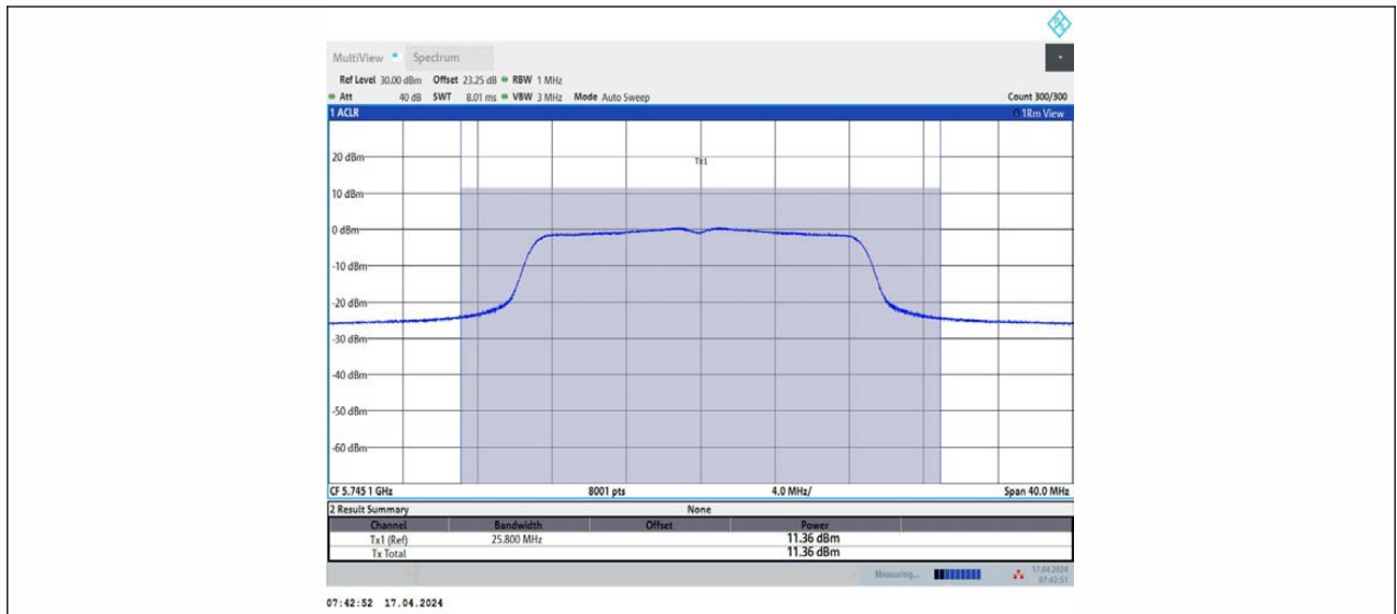
11N20MIMO_Ant2_5745
