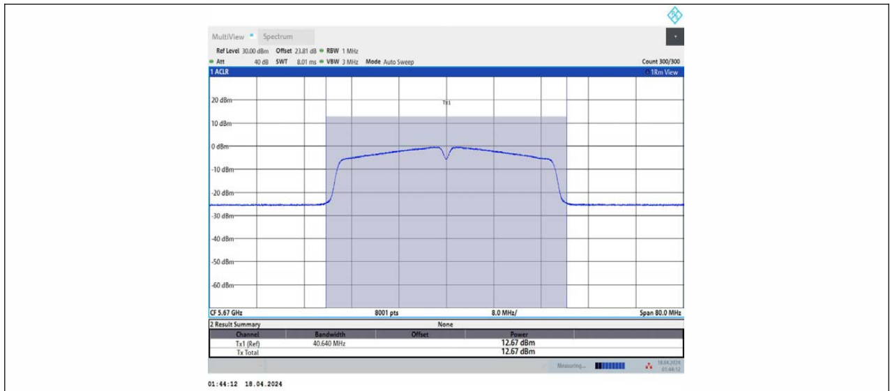
11AC40MIMO_Ant2_5670
