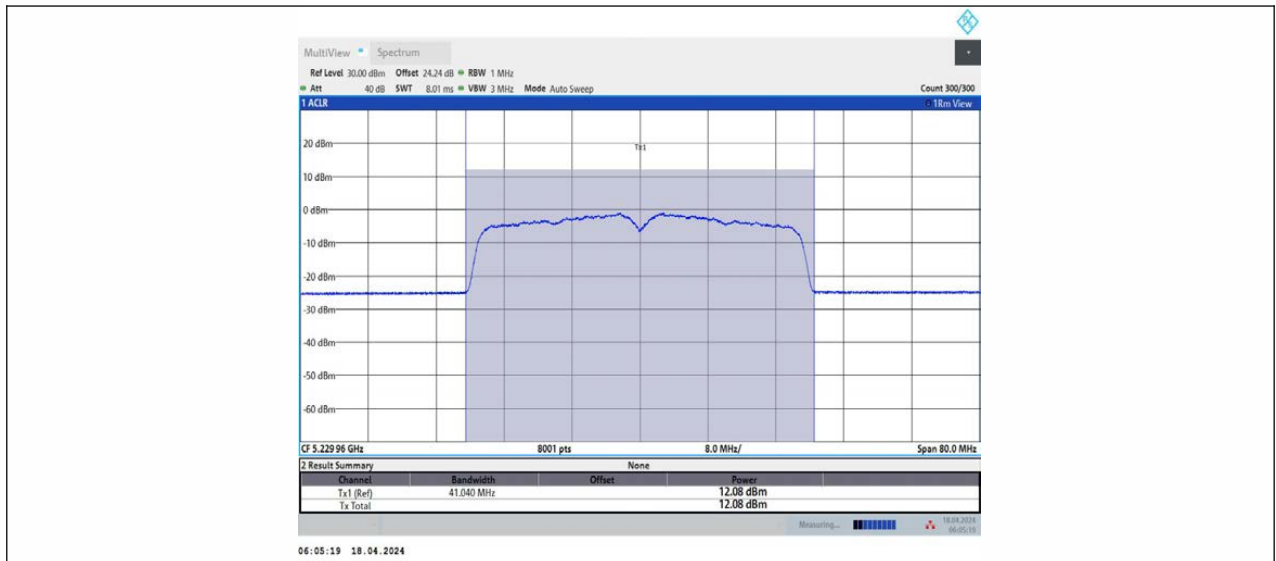
11AX40MIMO_Ant2_5230
