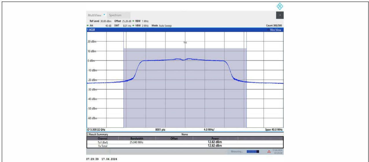
11N20MIMO_Ant2_5500
