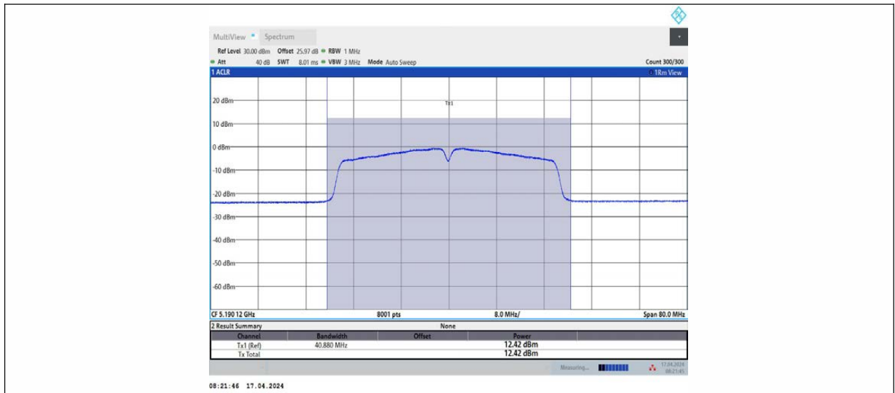
11N40MIMO_Ant2_5190
