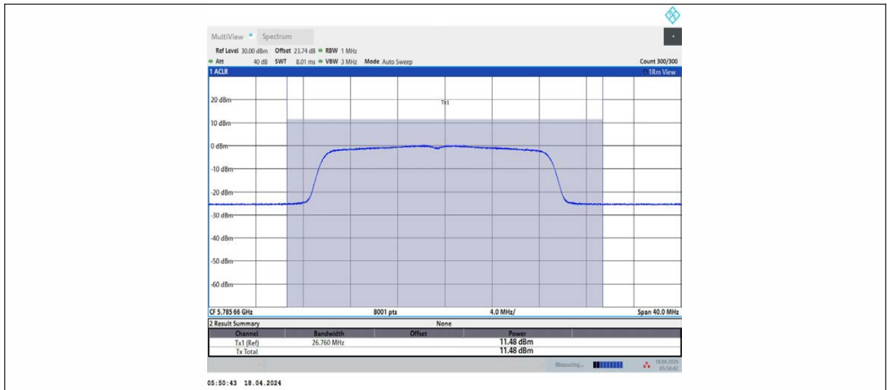
11AX20MIMO_Ant2_5785
