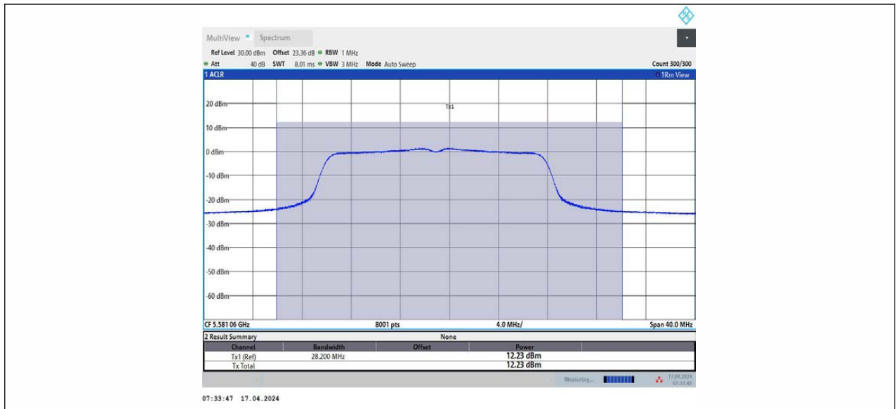
11N20MIMO_Ant2_5580
