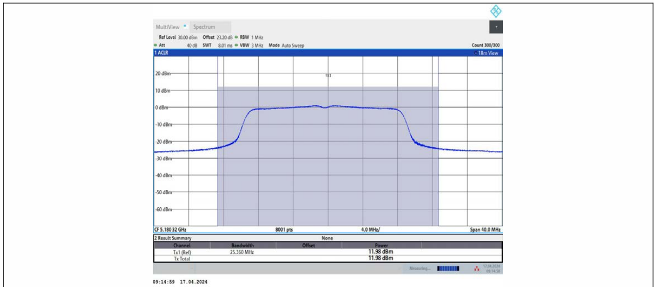
11AC20MIMO_Ant2_5180
