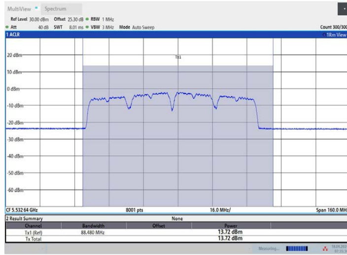
11AX80MIMO_Ant2_5530
