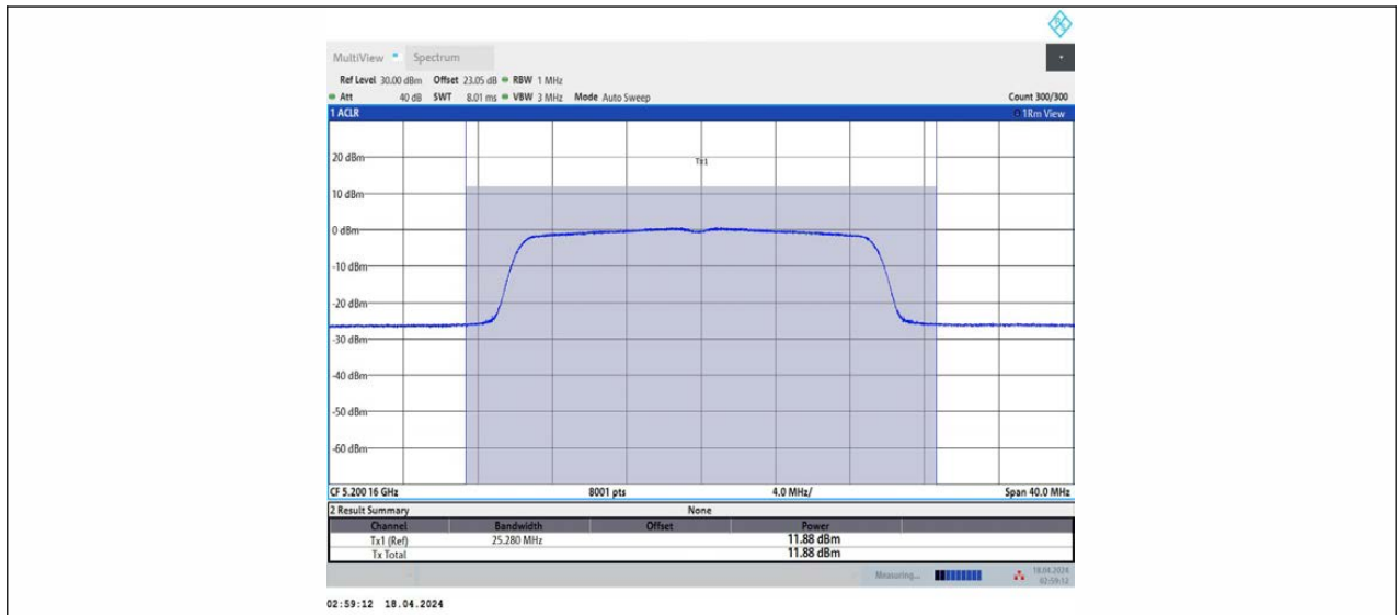
11AX20MIMO_Ant2_5200
