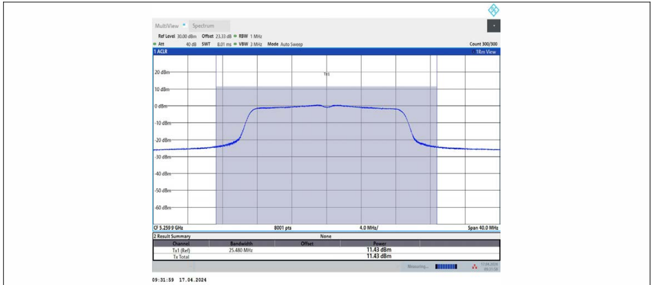
11AC20MIMO_Ant2_5260
