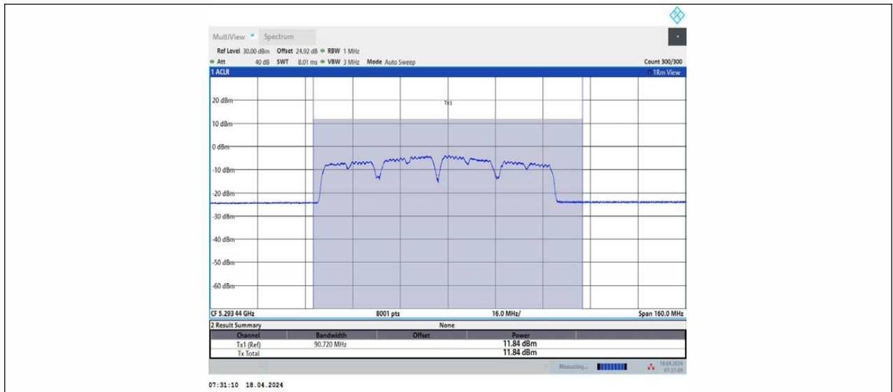
11AX80MIMO_Ant2_5290
