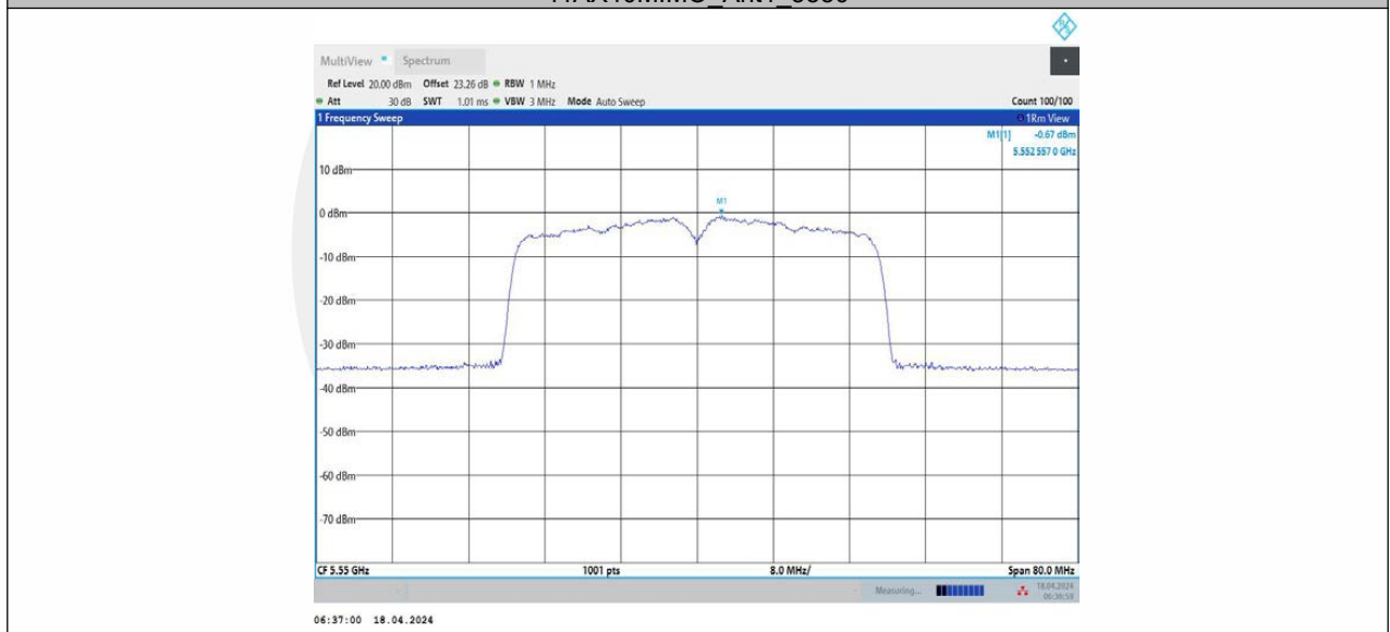
11AX40MIMO_Ant2_5550
