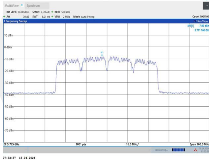
11AX80MIMO_Ant2_5775
