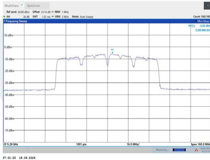
11AX80MIMO_Ant2_5290
