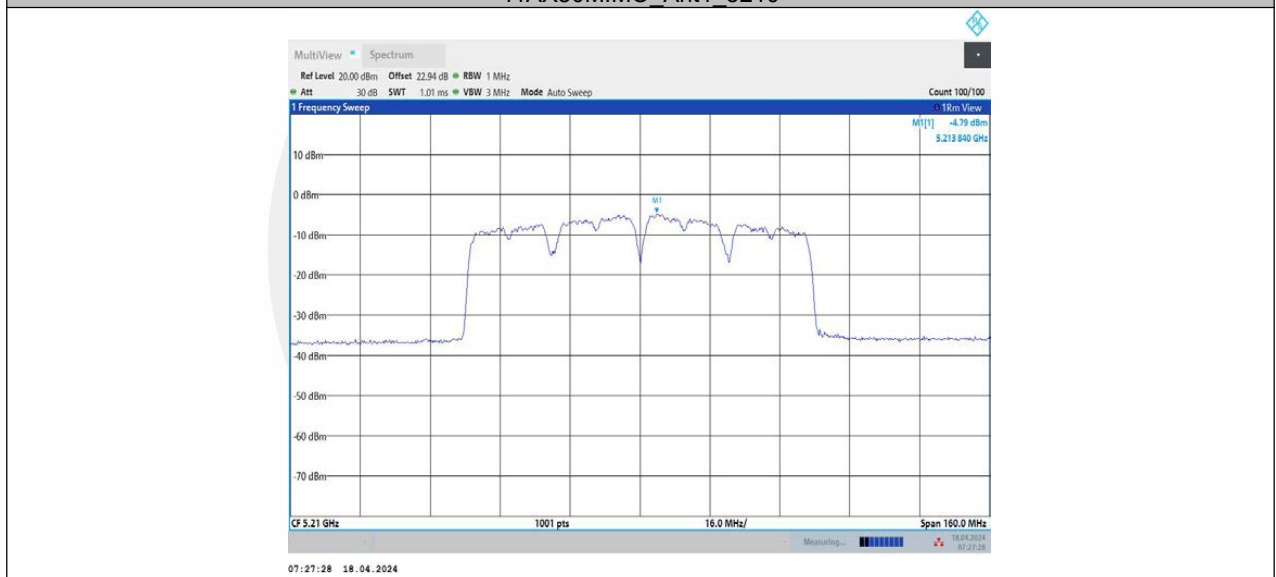
11AX80MIMO_Ant2_5210
