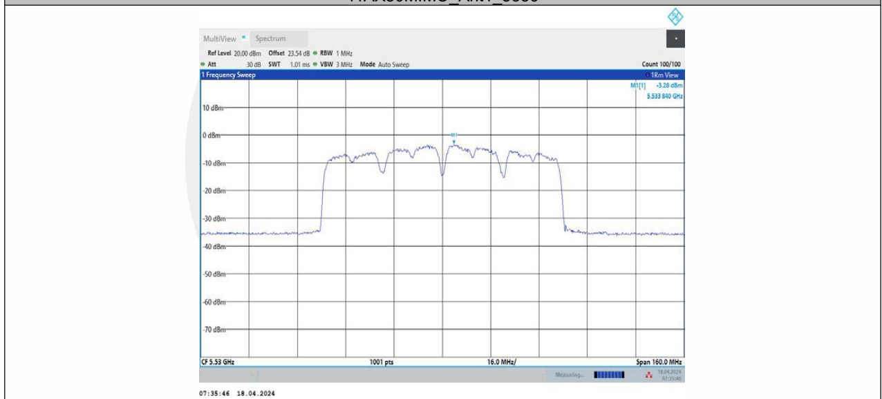
11AX80MIMO_Ant2_5530
