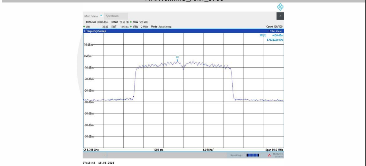
11AX40MIMO_Ant2_5795
