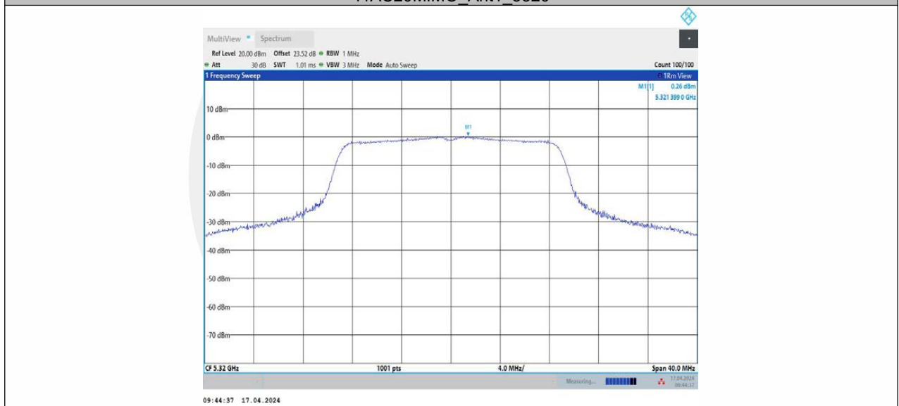
11AC20MIMO_Ant2_5320
