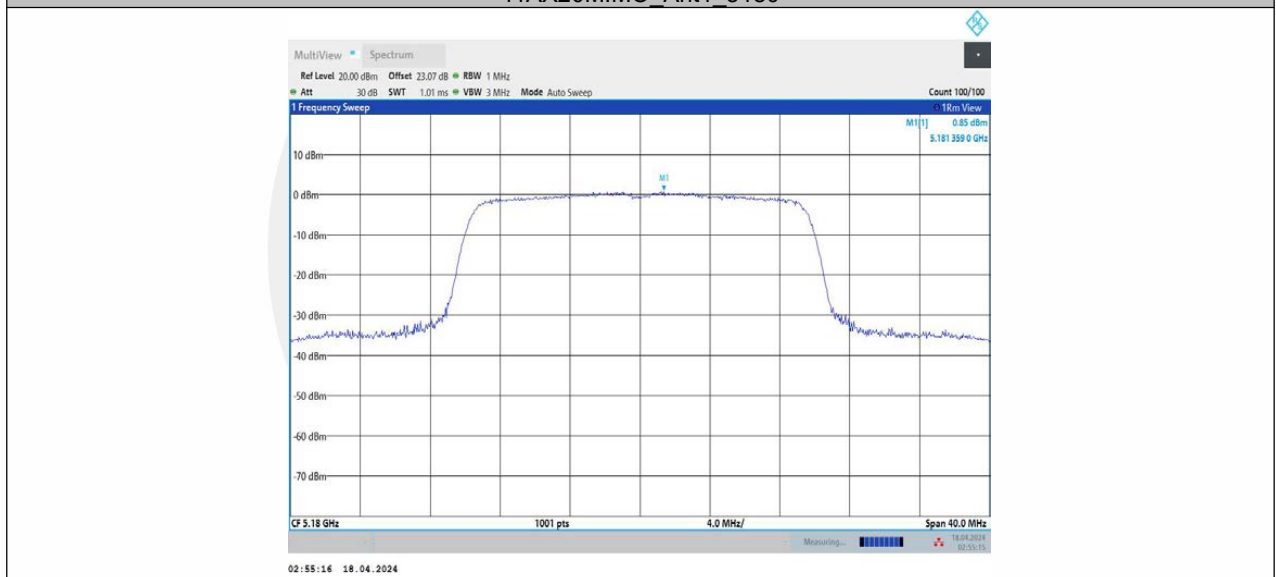
11AX20MIMO_Ant2_5180
