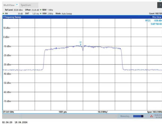
11AC80MIMO_Ant2_5610
