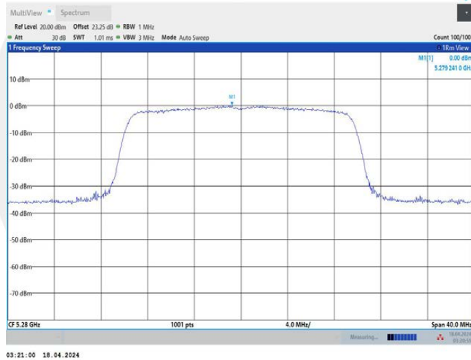
11AX20MIMO_Ant2_5280
