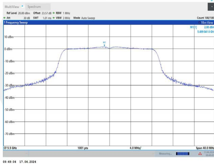
11AC20MIMO_Ant2_5500
