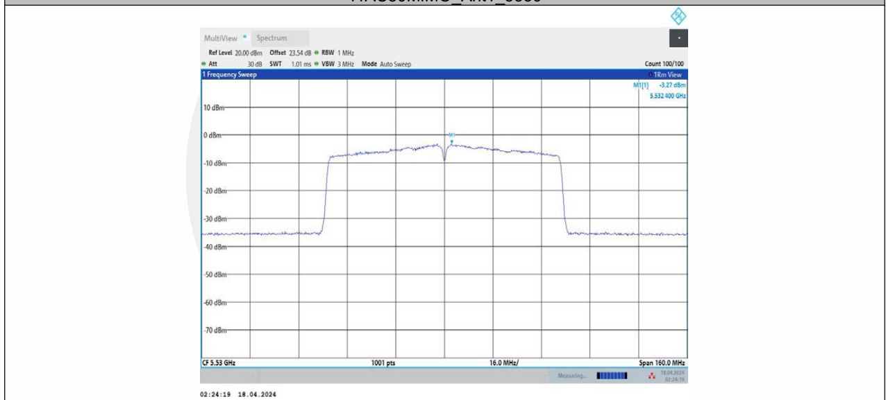
11AC80MIMO_Ant2_5530
