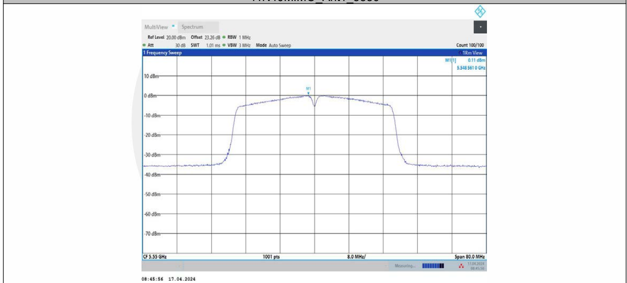
11N40MIMO_Ant2_5550
