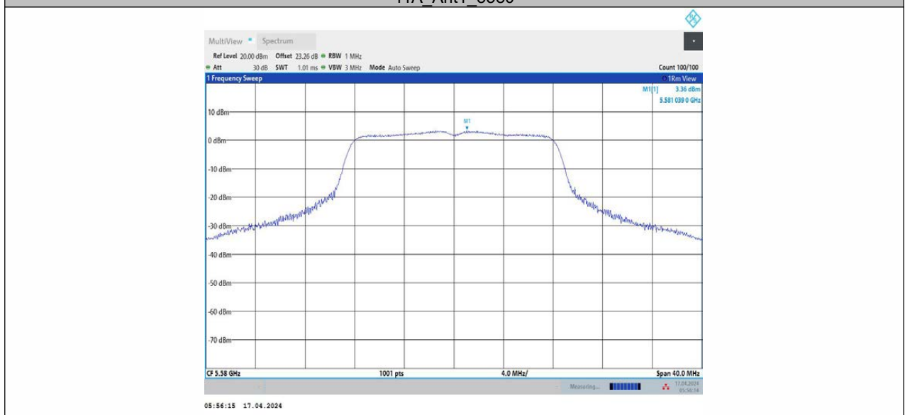
11A_Ant1_5580
