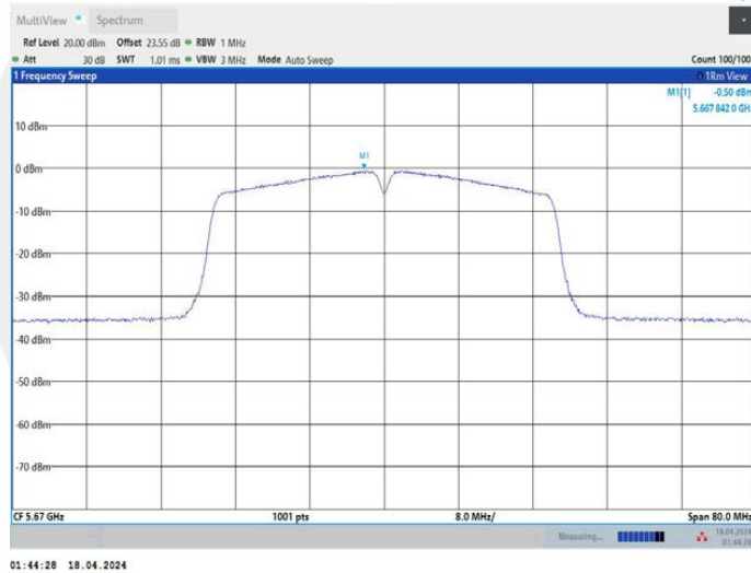
11AC40MIMO_Ant2_5670
