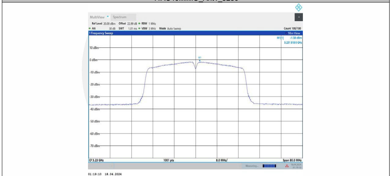
11AC40MIMO_Ant2_5230
