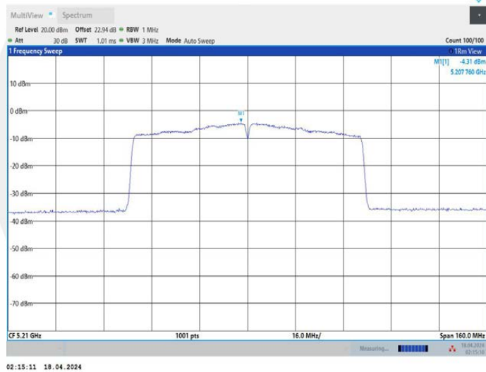
11AC80MIMO_Ant2_5210
