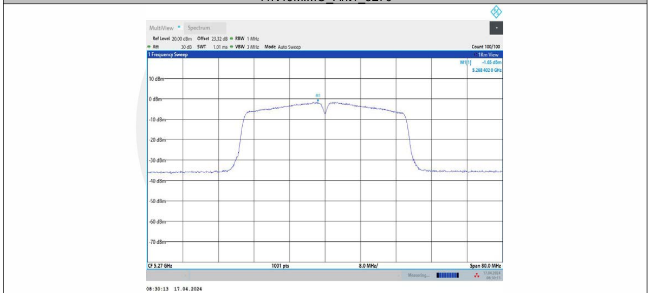
11N40MIMO_Ant2_5270
