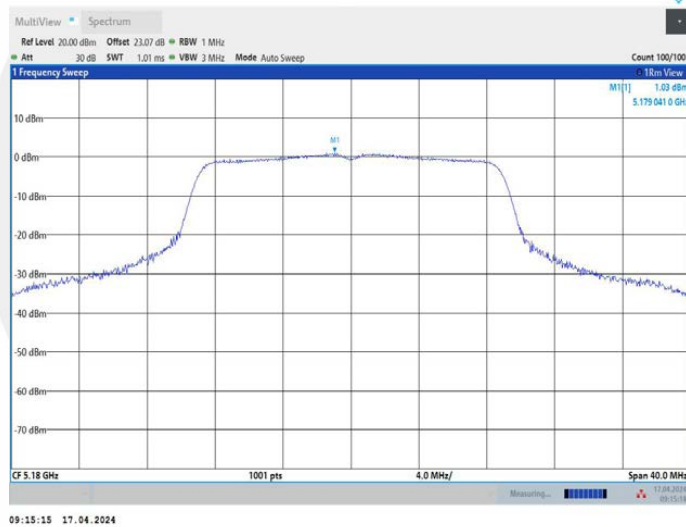
11AC20MIMO_Ant2_5180
