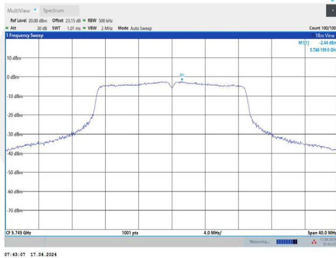
11N20MIMO_Ant2_5745
