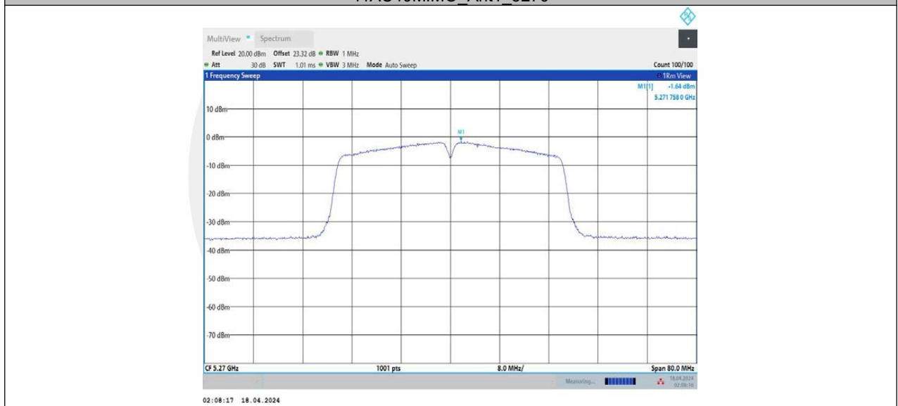
11AC40MIMO_Ant2_5270
