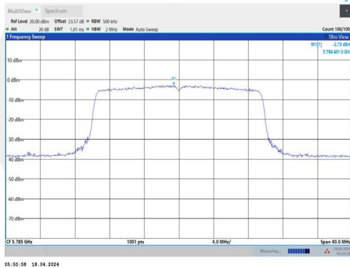
11AX20MIMO_Ant2_5785
