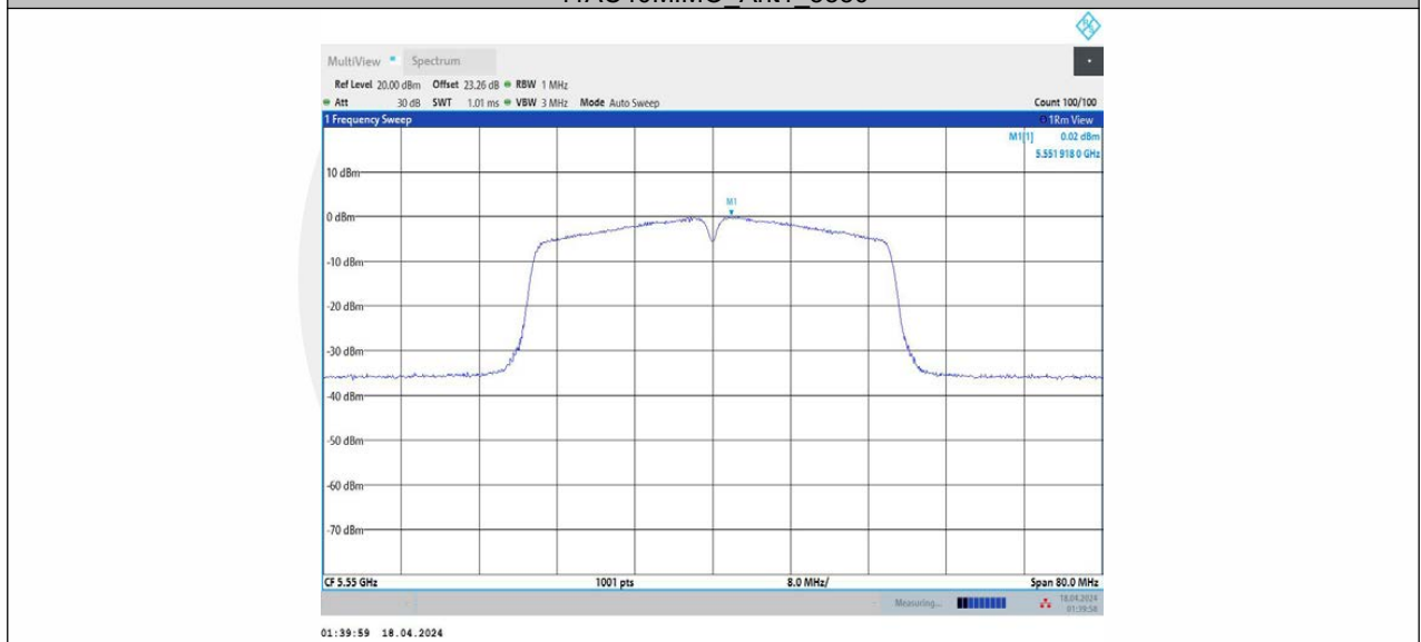
11AC40MIMO_Ant2_5550
