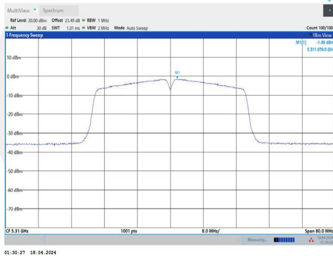
11AC40MIMO_Ant2_5310
