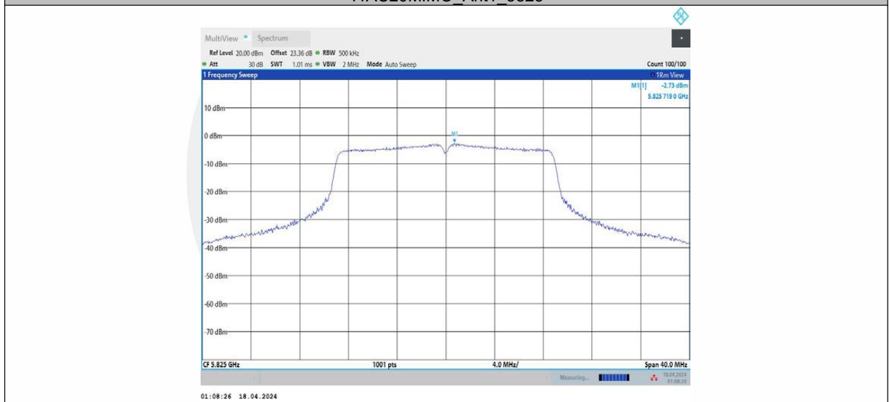
11AC20MIMO_Ant2_5825
