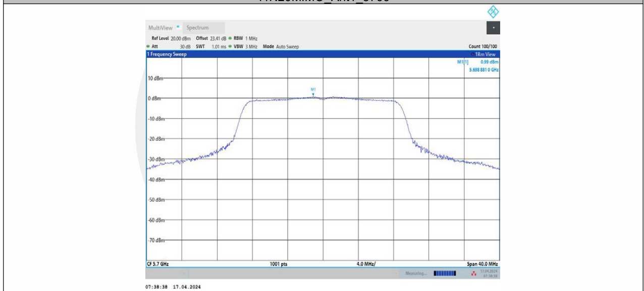
11N20MIMO_Ant2_5700
