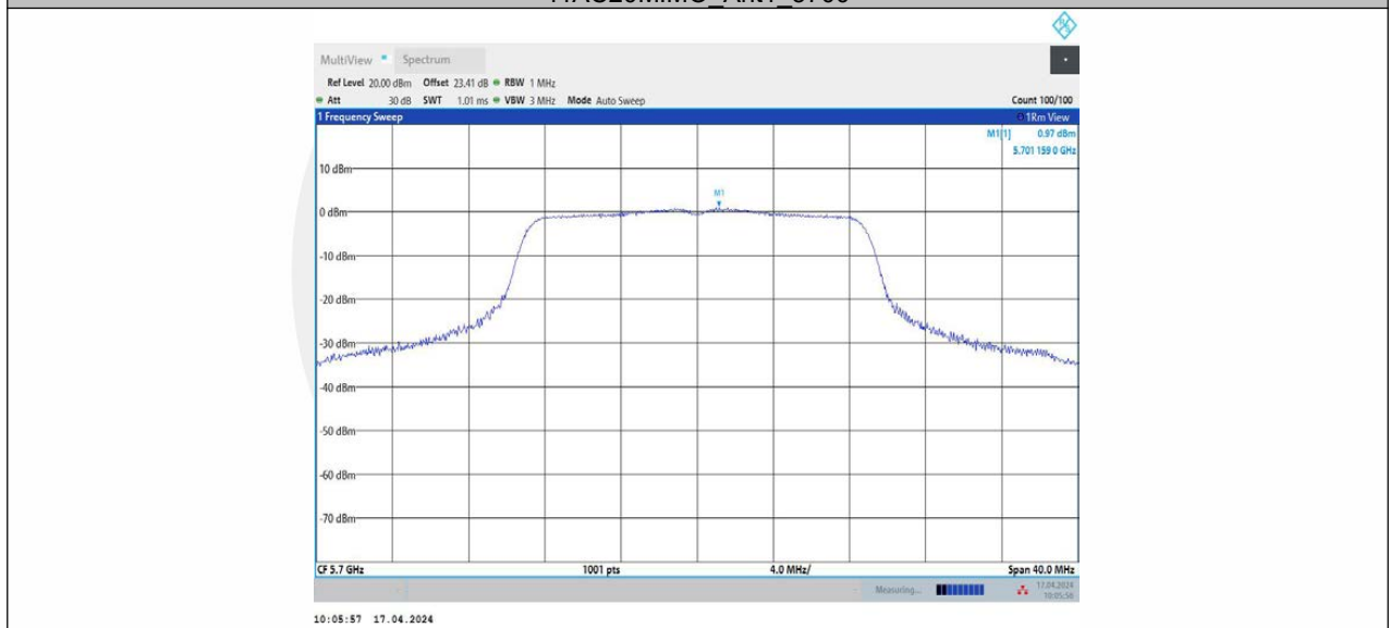
11AC20MIMO_Ant2_5700
