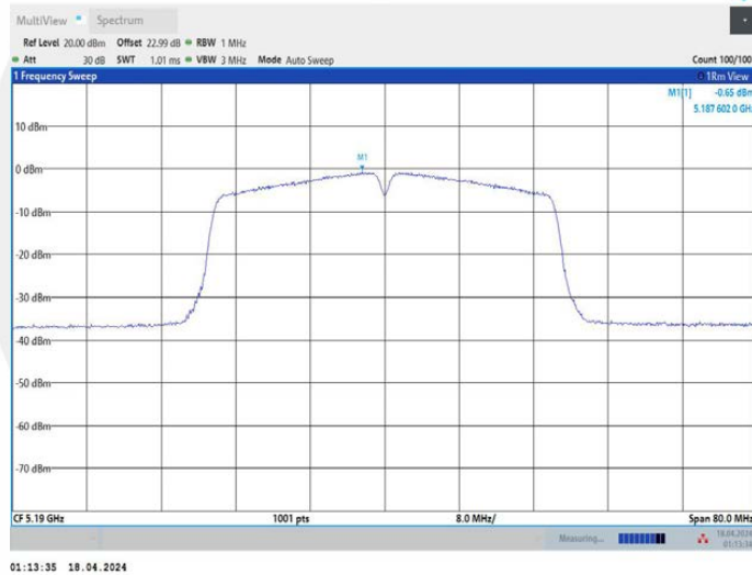
11AC40MIMO_Ant2_5190
