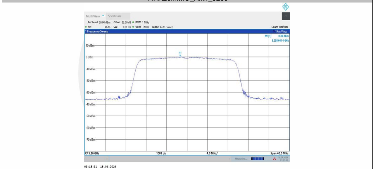
11AX20MIMO_Ant2_5260
