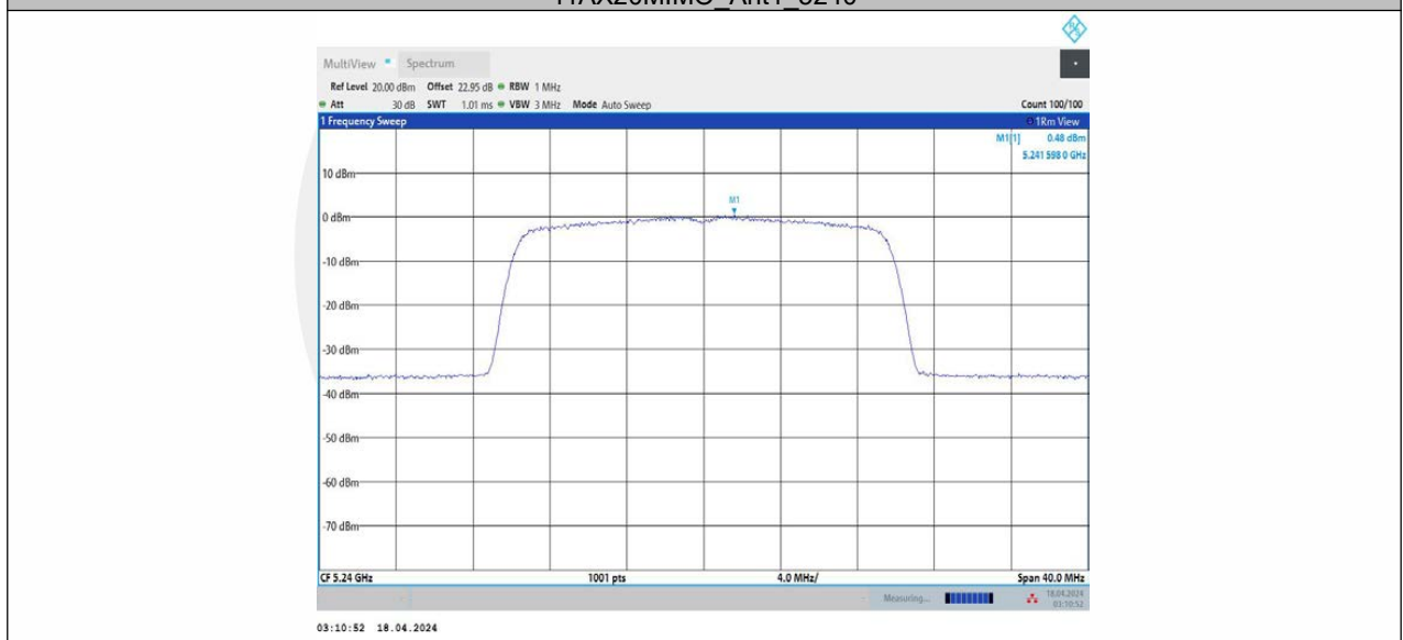
11AX20MIMO_Ant2_5240
