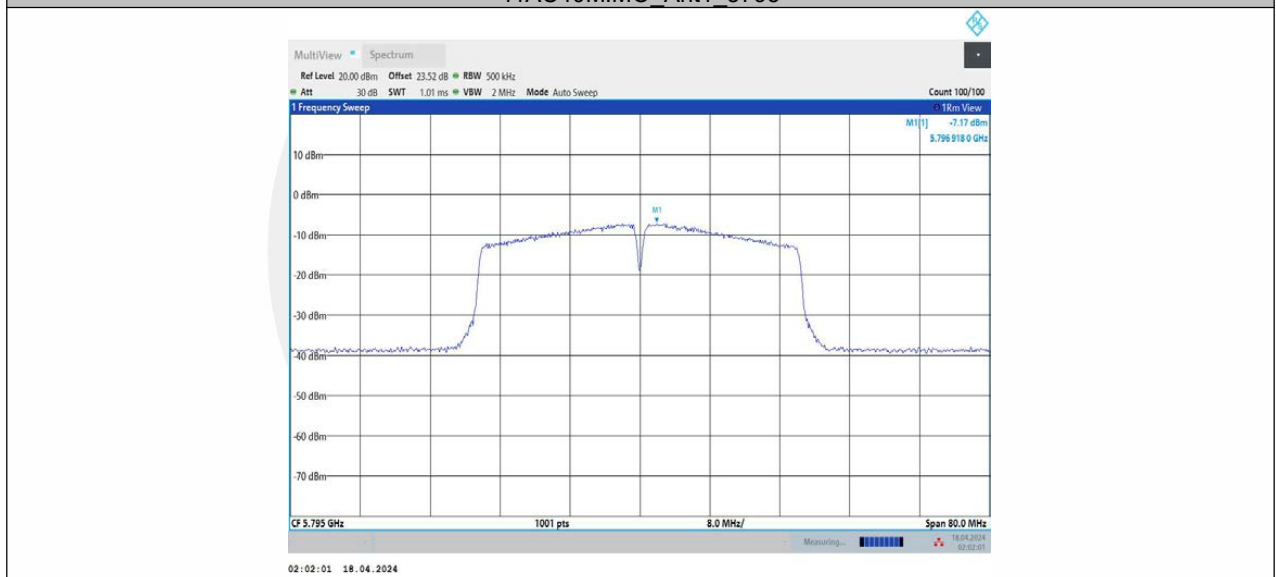
11AC40MIMO_Ant2_5795
