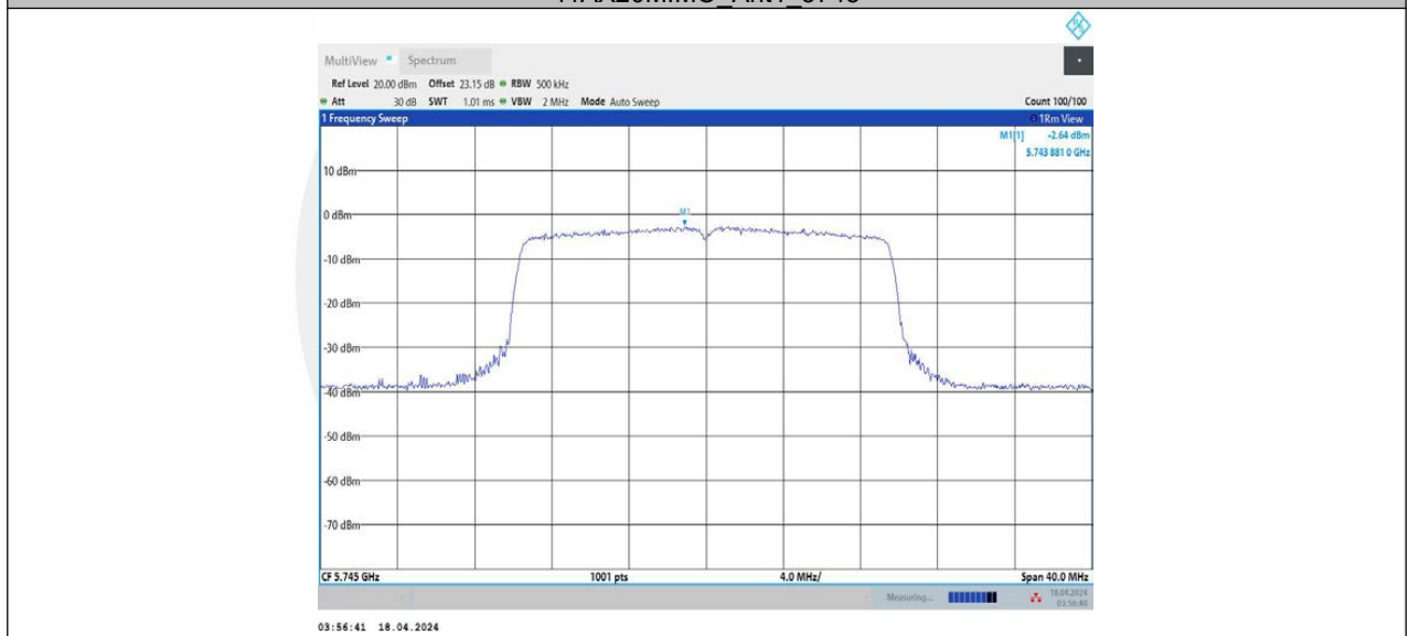
11AX20MIMO_Ant2_5745
