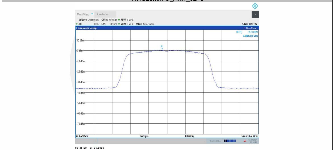
11AC20MIMO_Ant2_5240
