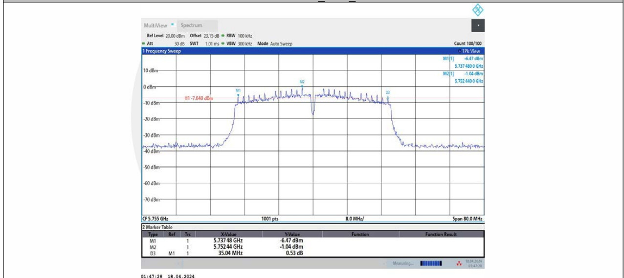
11AC40MIMO_Ant2_5755
