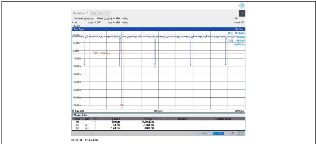
11A_Ant2_5320
