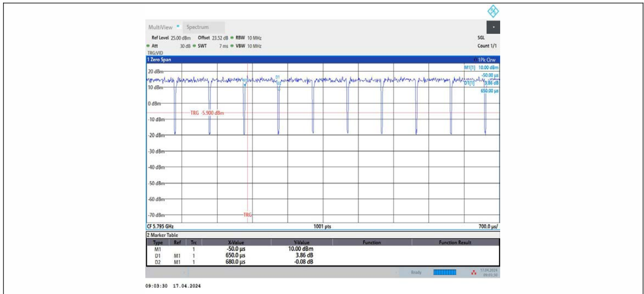
11N40MIMO_Ant2_5795
