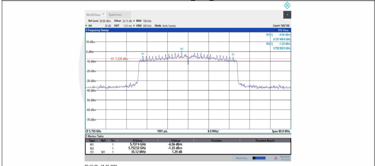
11AX40MIMO_Ant2_5755
