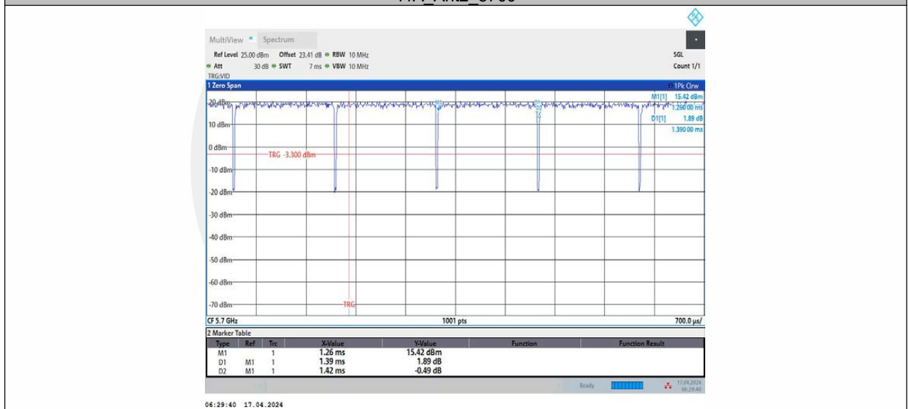
11A_Ant1_5745
