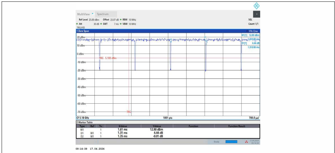
11AC20MIMO_Ant2_5180
