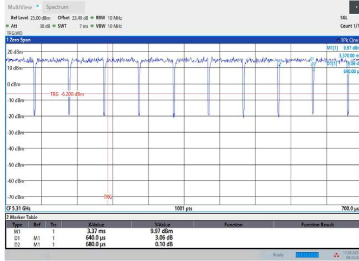
11N40MIMO_Ant2_5310
