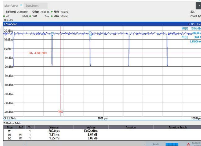
11AC20MIMO_Ant1_5745
