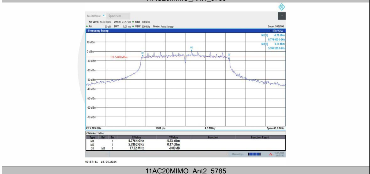
11AC20MIMO_Ant2_5785
