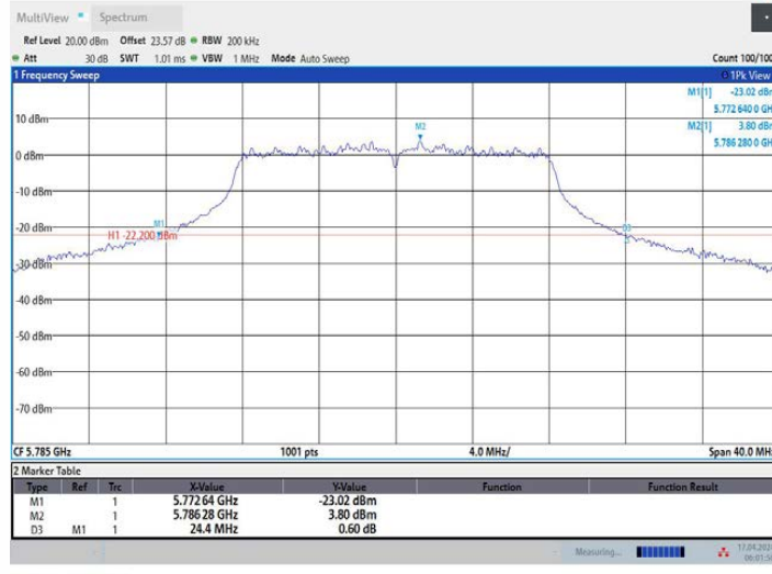
11A_Ant2_5785
