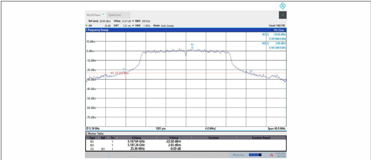
11AC20MIMO_Ant2_5180
