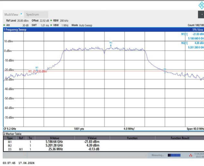
11A_Ant2_5200
