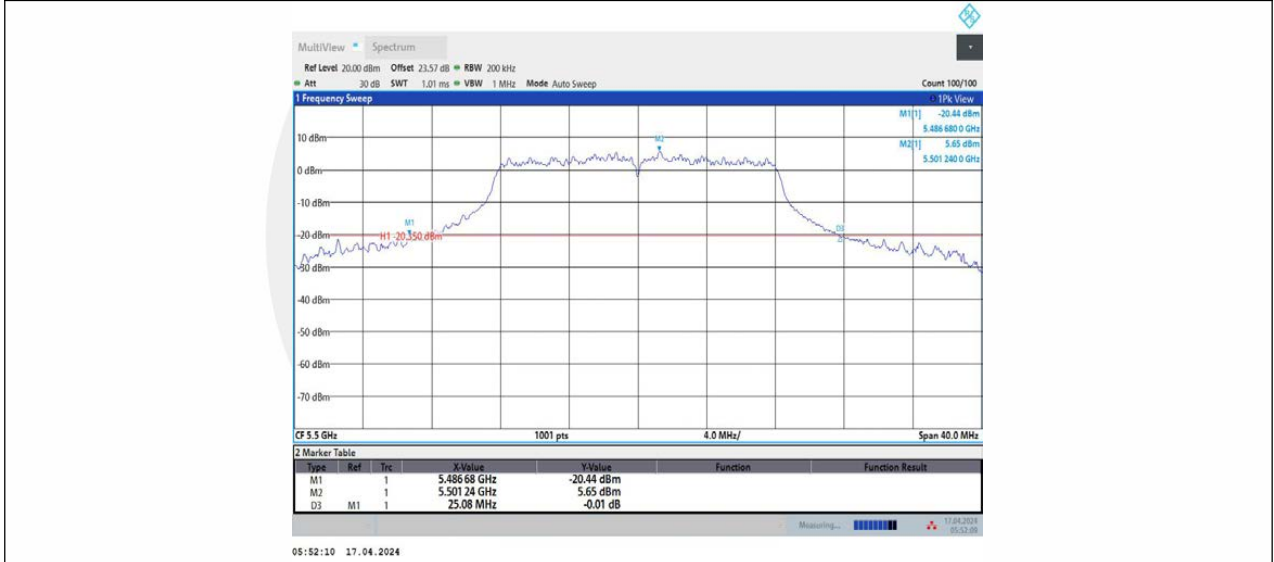
11A_Ant2_5500
