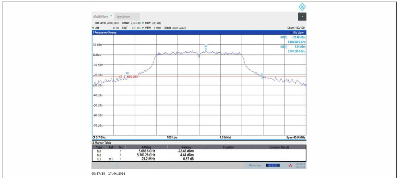
11A_Ant2_5700
