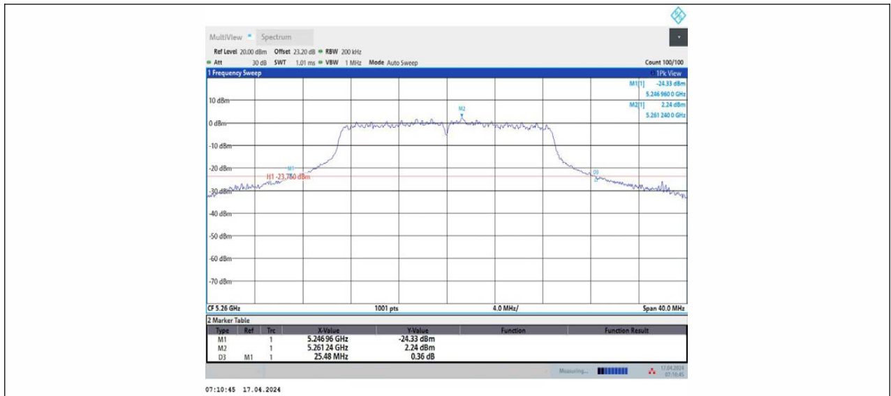
11N20MIMO_Ant2_5260
