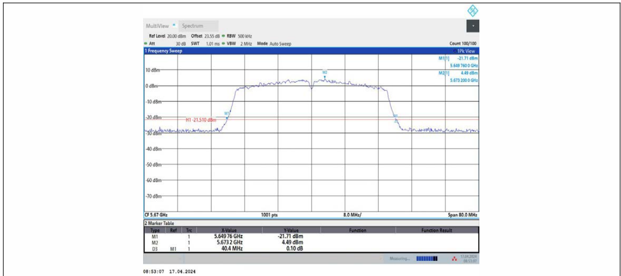
11N40MIMO_Ant2_5670
