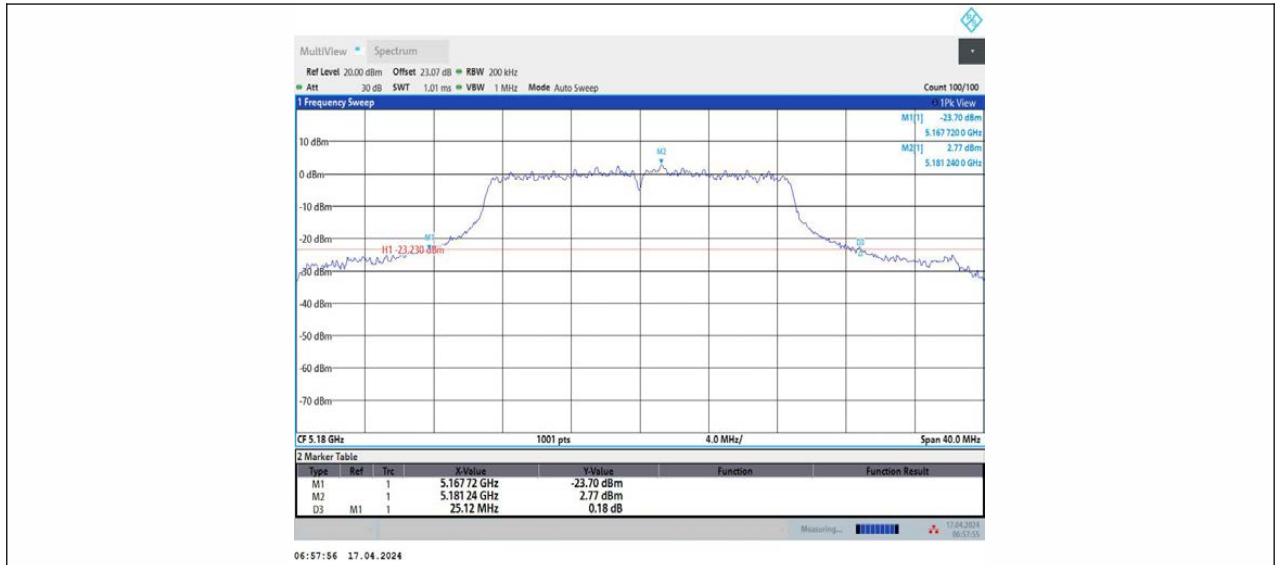
11N20MIMO_Ant2_5180
