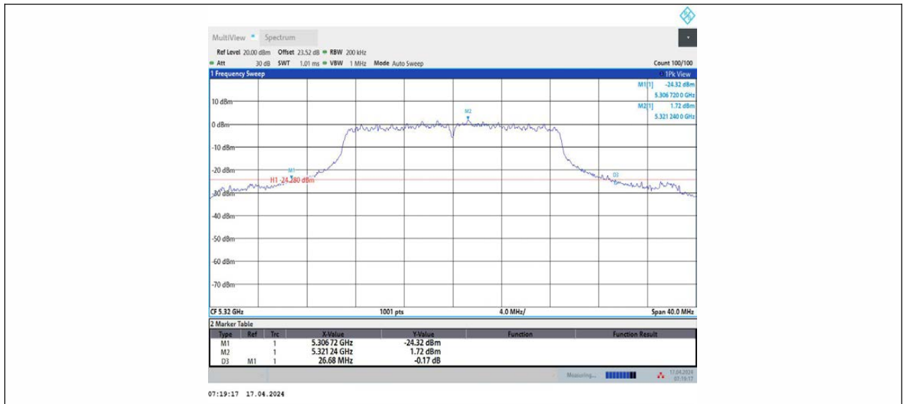
11N20MIMO_Ant2_5320
