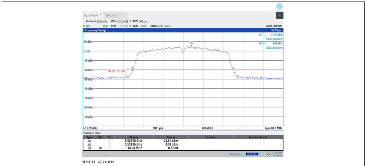
11N40MIMO_Ant2_5550
