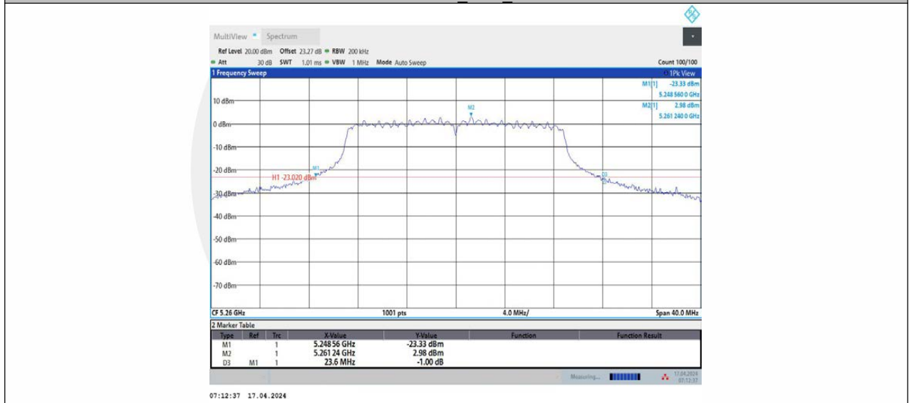
11N20MIMO_Ant1_5280
