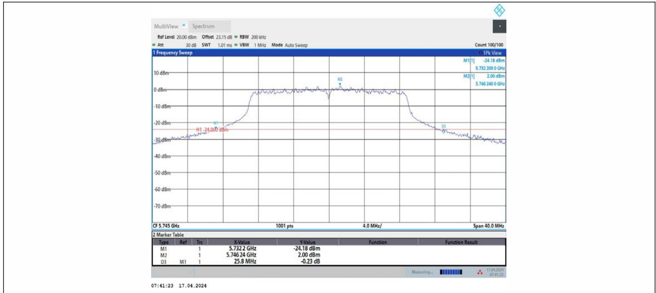
11N20MIMO_Ant2_5745
