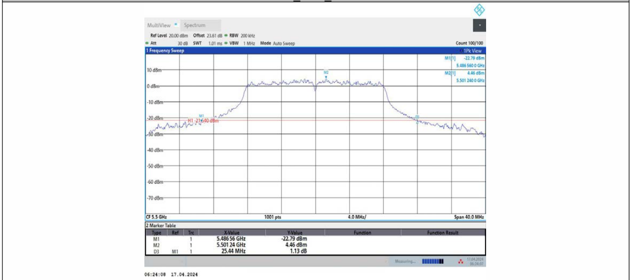
11A_Ant2_5500
