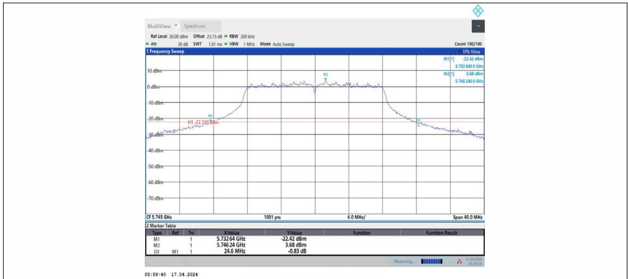
11A_Ant2_5745
