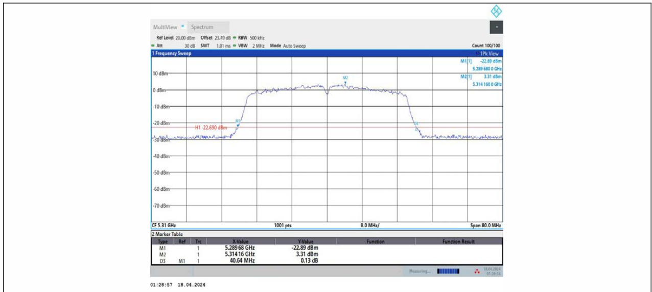
11AC40MIMO_Ant2_5310
