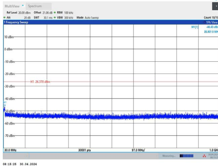
11AX20MIMO_Ant1_2437_30~1000
