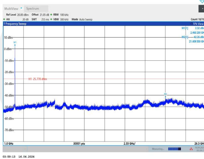
11N40MIMO_Ant1_2422_0~Reference
