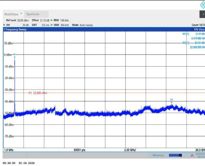
11AX40MIMO_Ant2_2422_0~Reference
