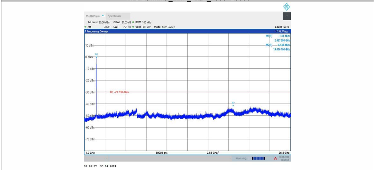
11AX20MIMO_Ant2_2462_1000~26500
