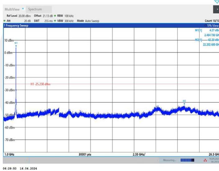
11N40MIMO_Ant2_2452_0~Reference
