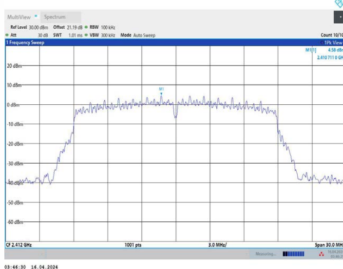
11N20MIMO_Ant2_2412_0~Reference
