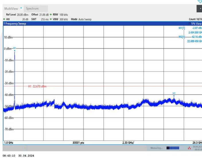
11AX40MIMO_Ant2_2437_0~Reference
