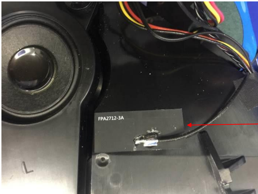
WiFi Antenna2
