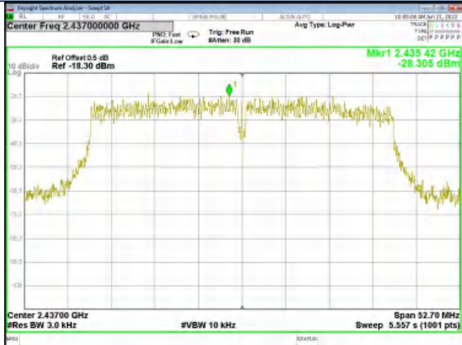
802.11n40 2437 MHz
