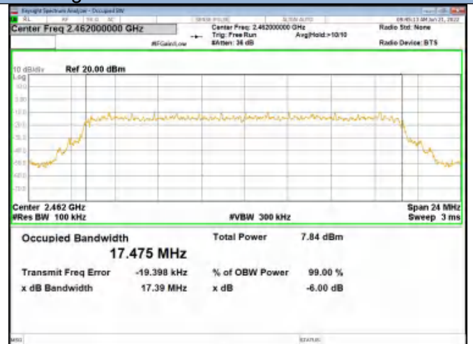
802.11g 2462 MHz
