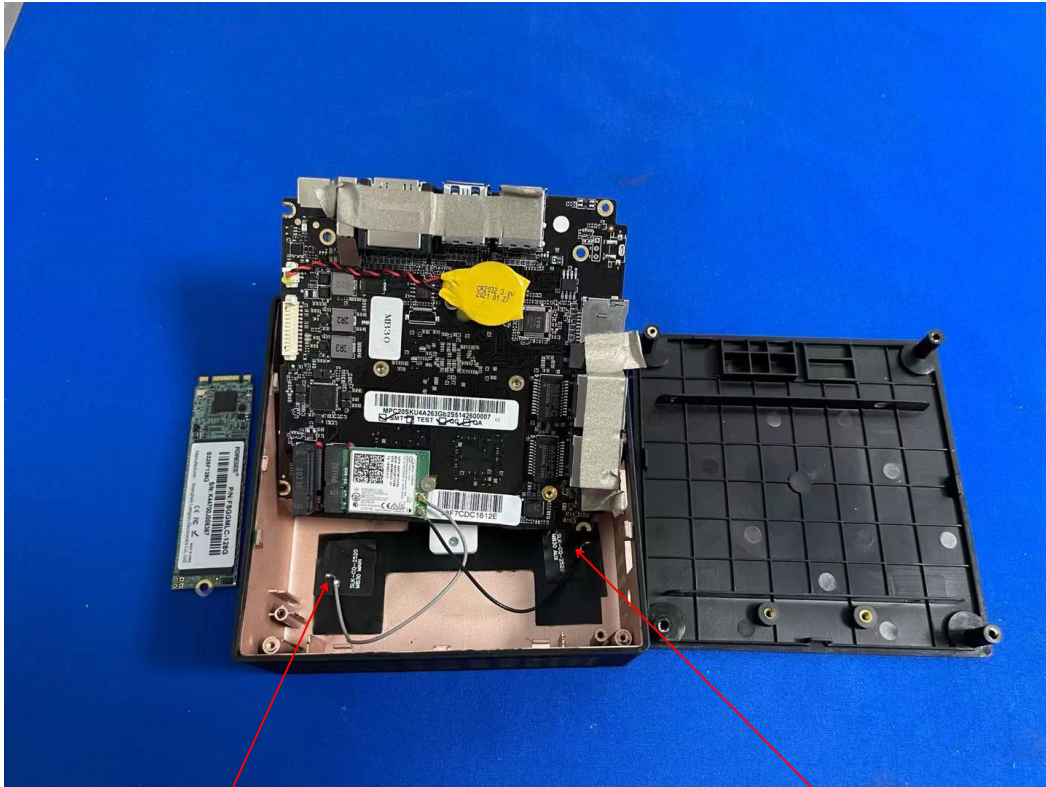
BT:Antenna
