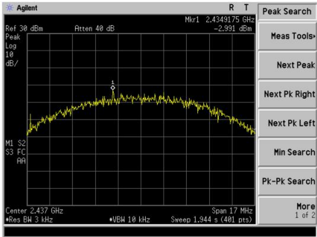
802.11b-2437MHz
