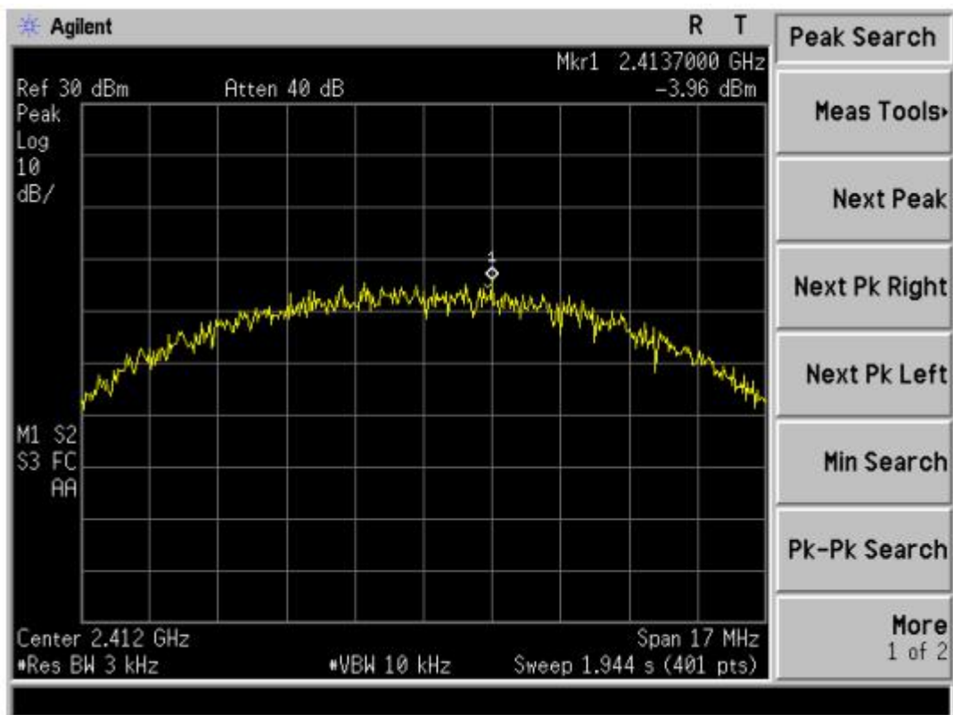
802.11b-2412MHz
