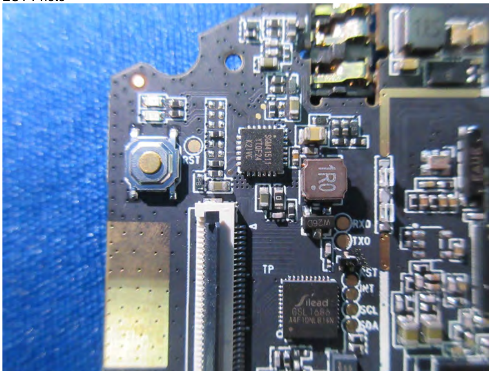
(40) EUT Photo
