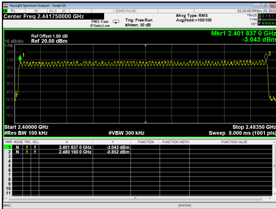
\pi/4 -DQPSK
