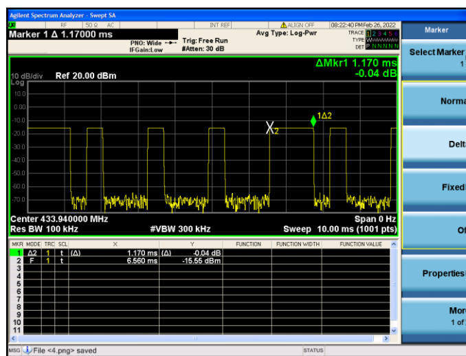
(Time per burst: 1.170\text{ms} \times 19\text{pcs} )
