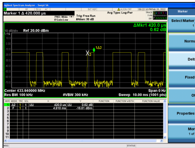
(Time per burst: 0.420\text{ms} \times 6\text{pcs} )
