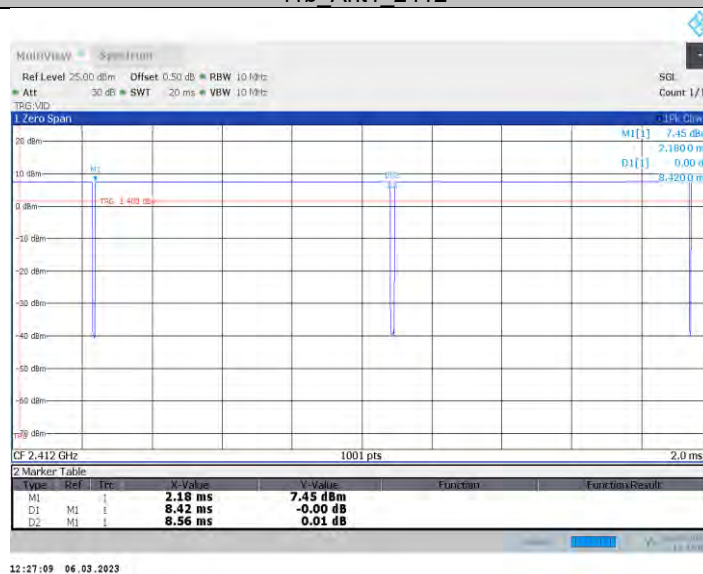
11b_Ant1_2412
