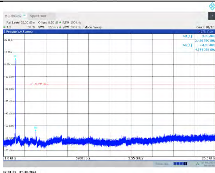
11b Ant0 2437 1000~26500
