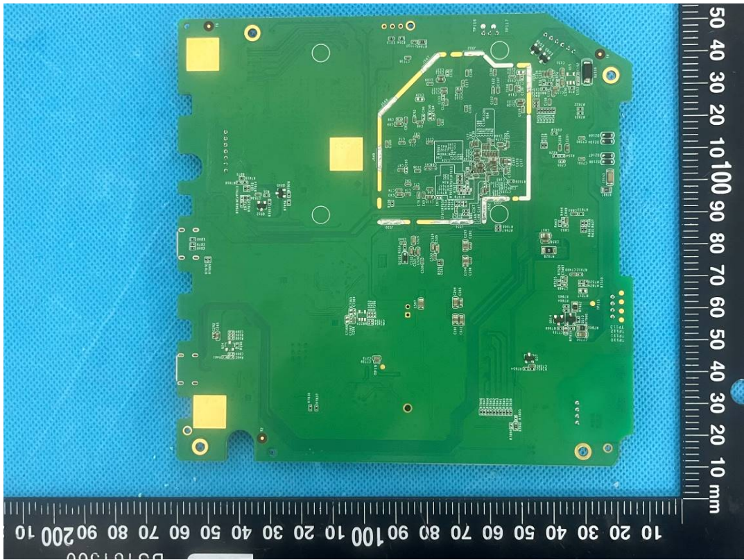
BT/WiFi Antenna
