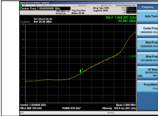
Band2-20MHz-16QAM-18700-1RB#0
