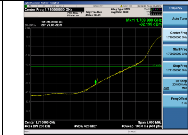
Band4-20MHz-QPSK-20050-1RB#0
