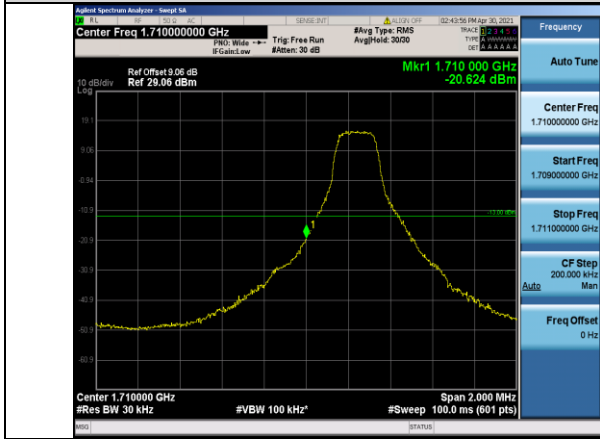
Band4-3MHz-QPSK-19965-1RB#0
