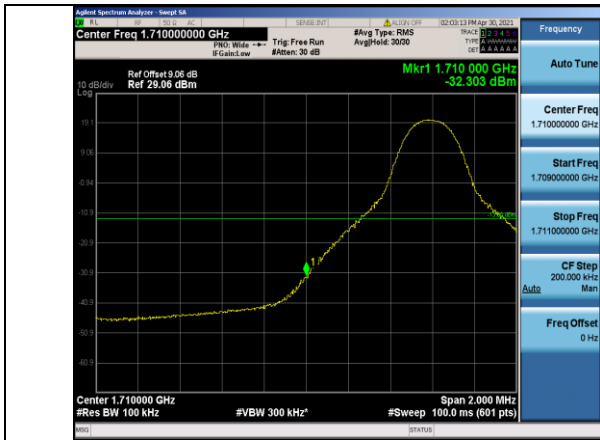
Band4-10MHz-QPSK-20000-1RB#0
