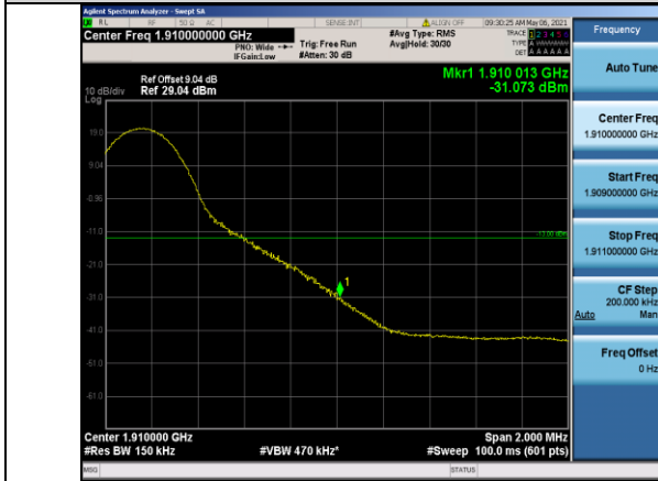
Band2-15MHz-16QAM-19125-1RB#74
