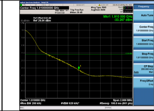
Band2-20MHz-16QAM-19100-1RB#99
