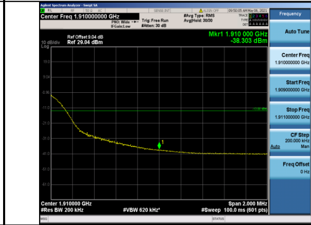
Band2-20MHz-16QAM-19100-100RB#0
