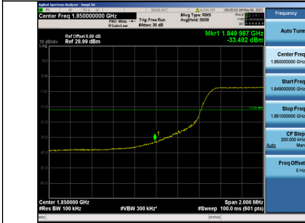
Band2-10MHz-QPSK-18650-50RB#0
