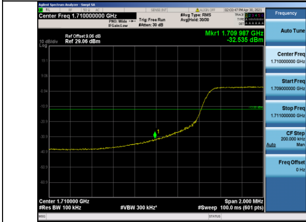
Band4-10MHz-QPSK-20000-50RB#0
