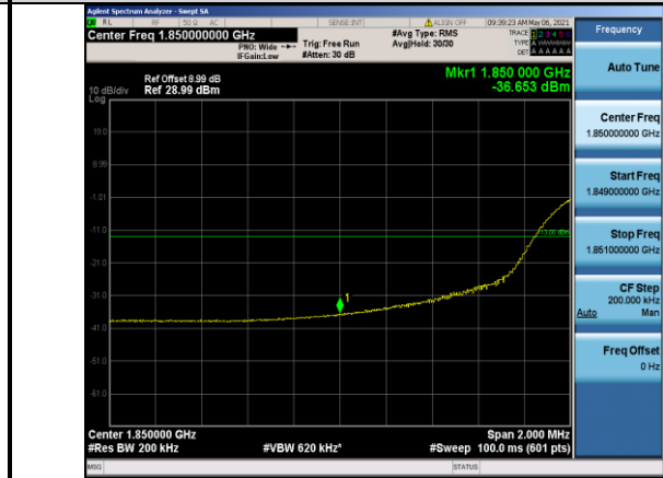
Band2-20MHz-QPSK-18700-100RB#0
