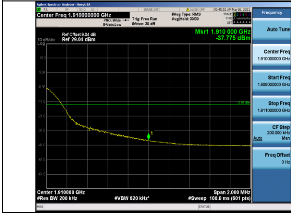
Band2-20MHz-QPSK-19100-100RB#0
