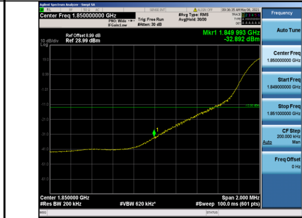
Band2-20MHz-QPSK-18700-1RB#0
