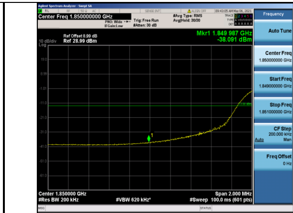
Band2-20MHz-16QAM-18700-100RB#0
