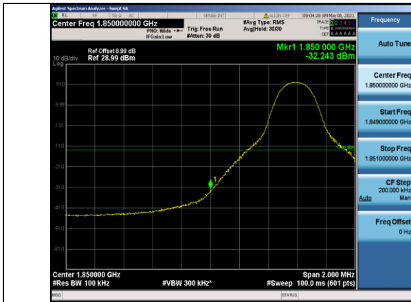
Band2-10MHz-QPSK-18650-1RB#0
