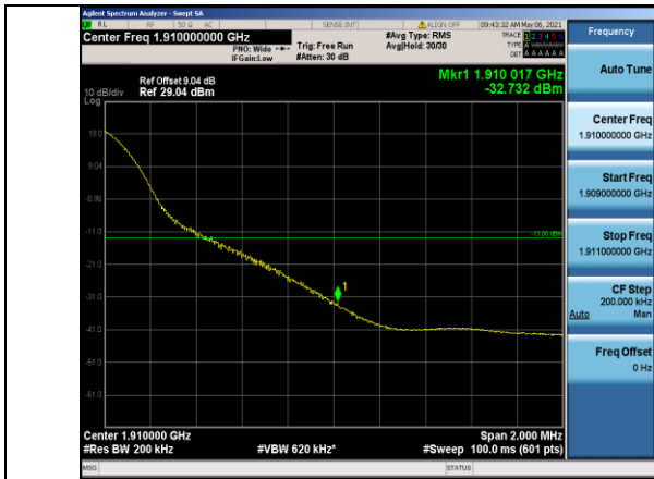
Band2-20MHz-QPSK-19100-1RB#99
