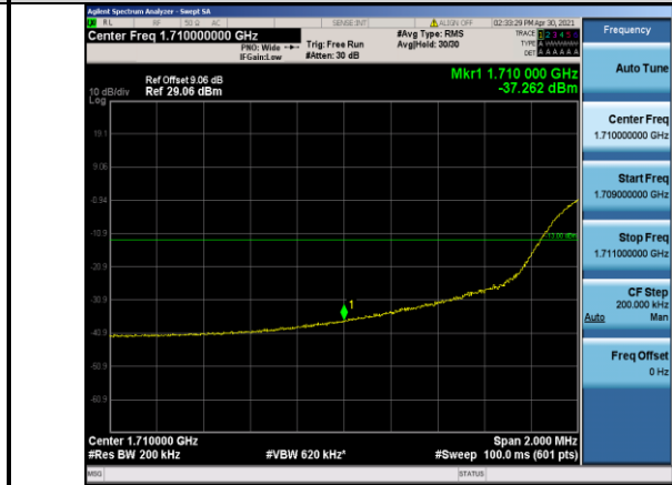
Band4-20MHz-QPSK-20050-100RB#0
