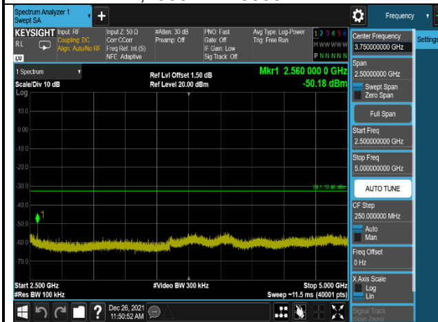
802.11n(HT40),2452MHz,Ant0,Plot 4,2500MHz~5000MHz
