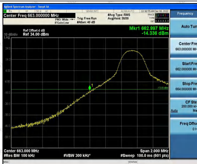
Band71-5MHz-QPSK-133147-1RB#24
