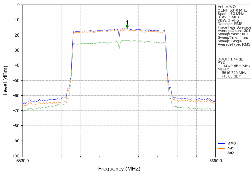
802.11ac(VHT80)_HCH_5610MHz_MIMO_NTNV
