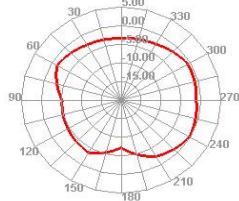
2450.000MHz E2
