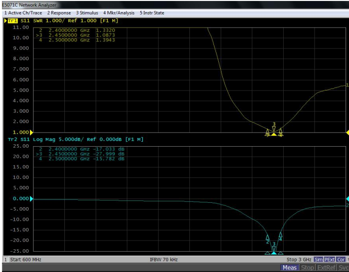
2450.000MHz H
