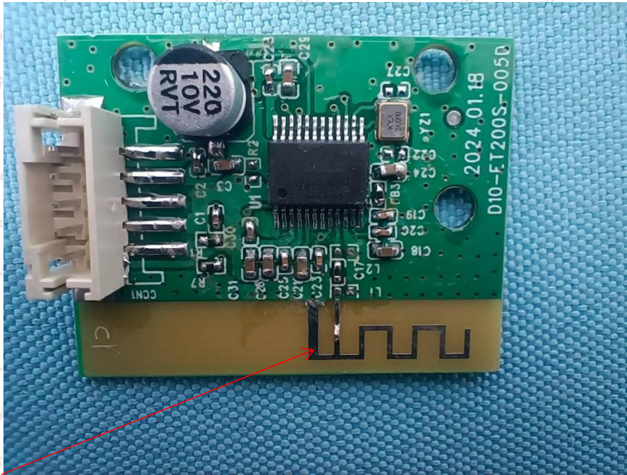
RX ANT
