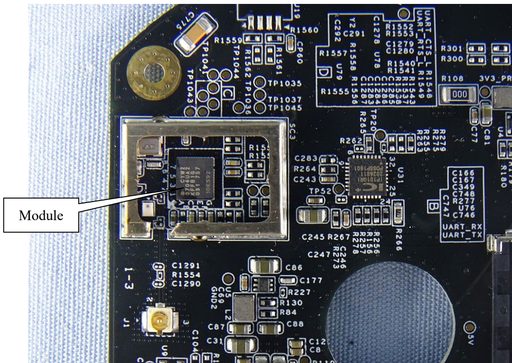
(10) EUT Photo
