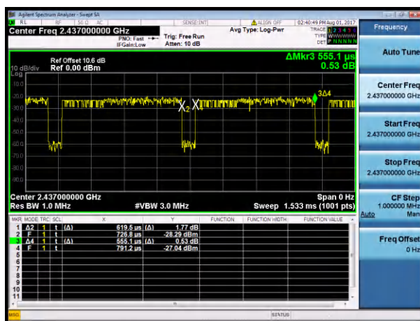
802.11n(20MHz)(2437MHz)
