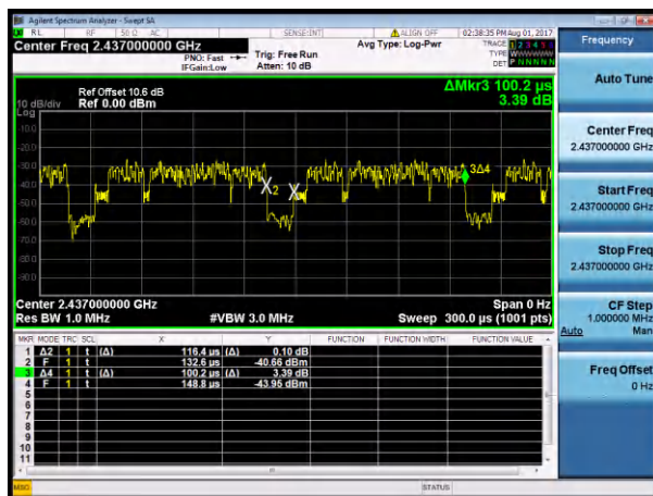
802.11n(20MHz)(2437MHz)
