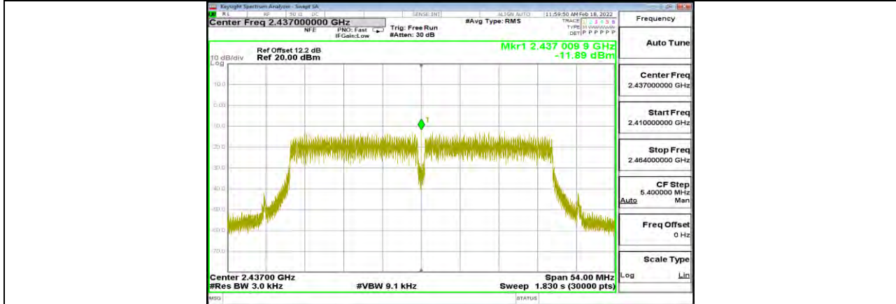
11N40SISO Ant1 2437
