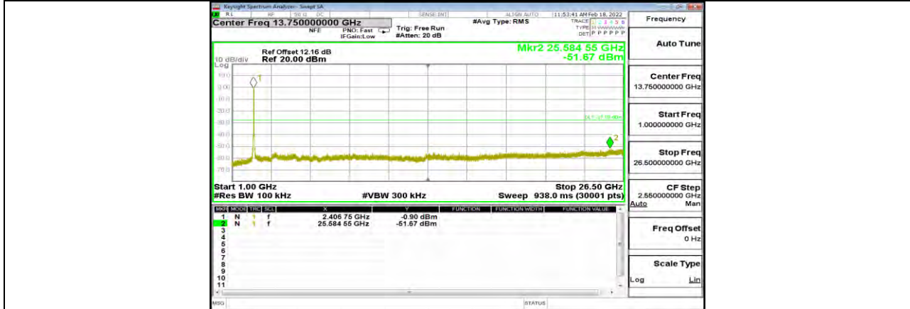
11N40SISO Ant1 2422 1000~26500
