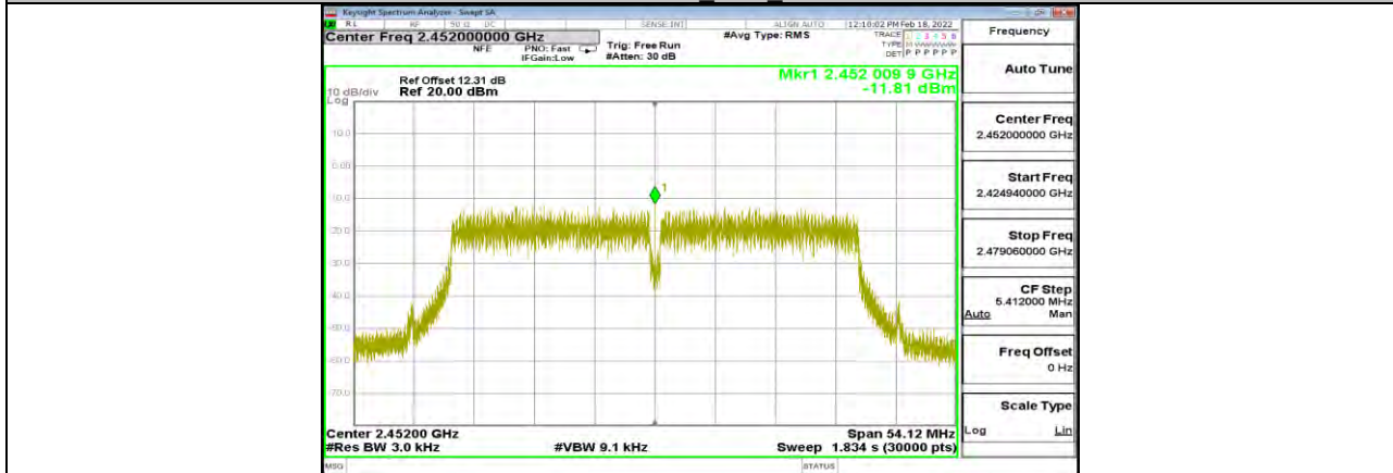
11N40SISO Ant1 2452
