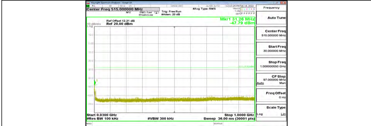
11N40SISO Ant1 2452 30~1000
